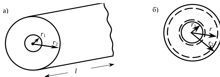
Рисунок 2.5 – Расчет напряженности электрического поля
