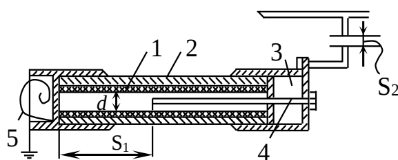
Рисунок 5.2 – Трубчатый разрядник
