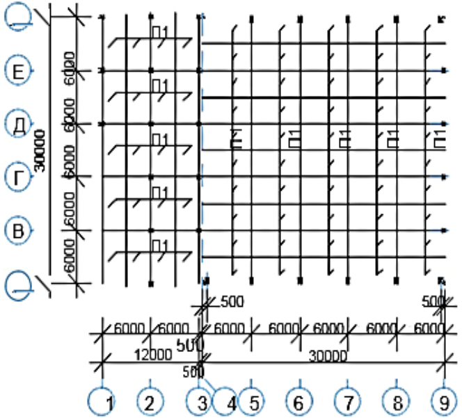
Рисунок 2.Схема расположения плит покрытия
