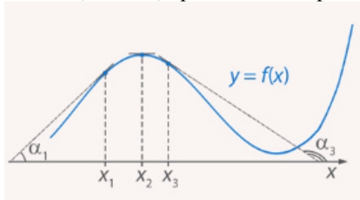
Угол наклона касательной в точке x_3
