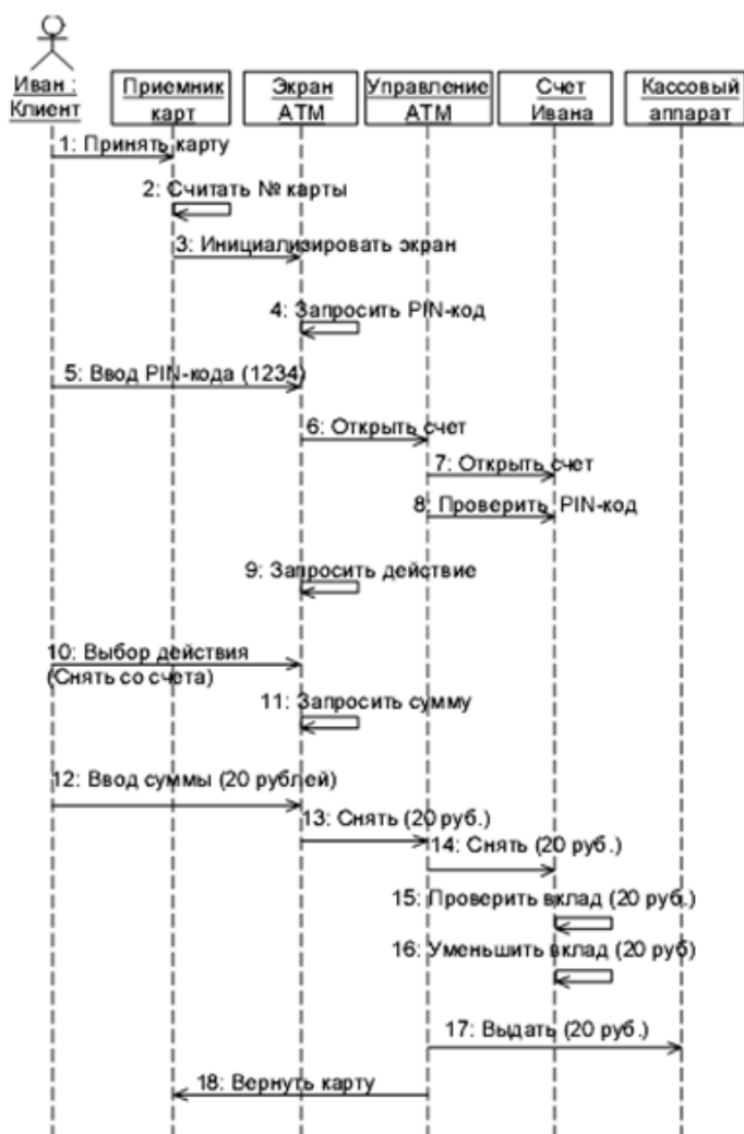
Рисунок 3.7 - Пример диаграммы последовательности
