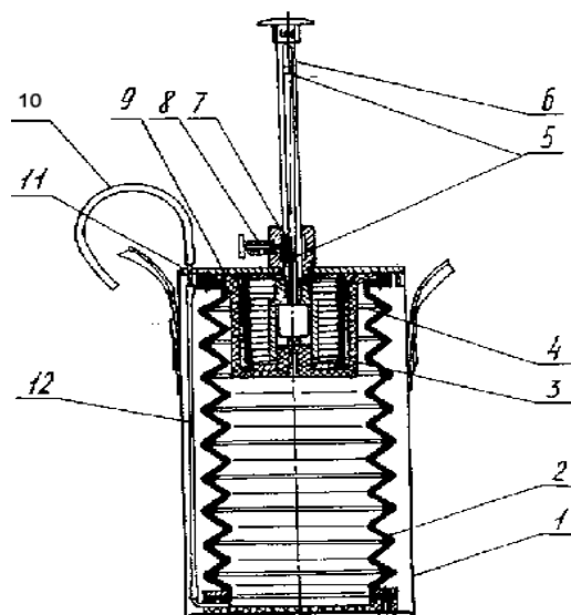
Рисунок 3.1– Устройство газоанализатора УГ-2: 1 – корпус, 2 – сильфон, 3 – пружина, 4 – кольцо распорное, 5 – канавка с двумя углублениями, 6 – шток, 7 – втулка, 8 – фиксатор, 9 – плата, 10 – трубка резиновая, 11 – штуцер, 12 – трубка резиновая
