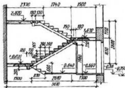
Рис. 3. Лестница из сборных мелкогазмерных элементов
