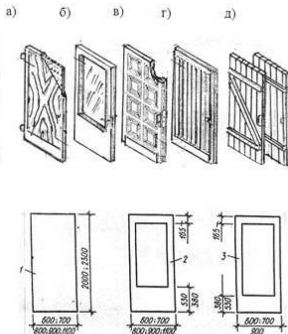
Рисунок 2. Полотна деревянных дверей: а- щитовое глухое; б- остекленное; в- филленчатое; г – филленчатое повышенной звукоизоляции; д- плотничные двери на планках и шпонках; 1 – глухие; 2 – остекленные; 3 – с качающимися полотнами.
