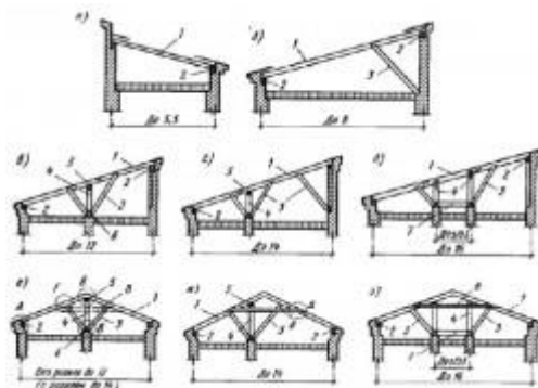
Рис. 3. Конструктивные схемы крыш из деревянных наслонных стропил (размеры даны в м): а—д - для односкатных крыш, е — з — для двускатных
