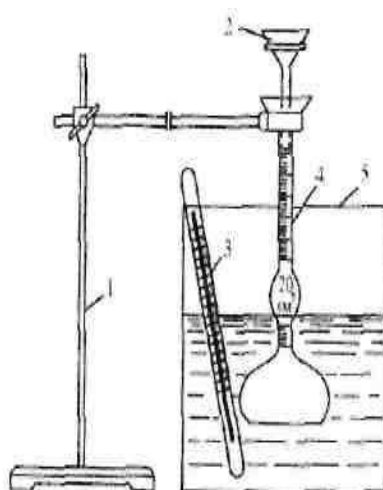
1 - штатив, 2 – воронка, 3 – термометр, 4 –объеммер, 5 – стеклянный сосуд
