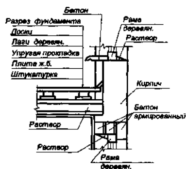
Междустажное перекрытие
