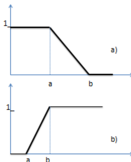
Рисунок 2 - Графики линейной Z-образной (a) и S-образной (b) функций принадлежности
