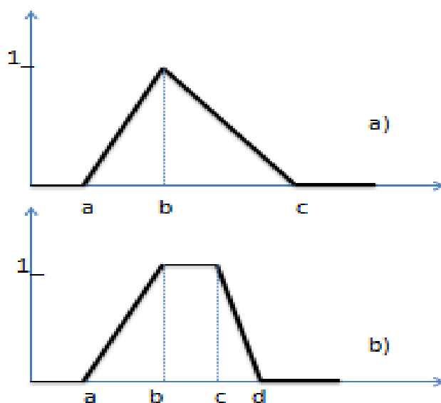
Рисунок 1 - Графики функций принадлежности треугольной (а), трапецевидной (b)
