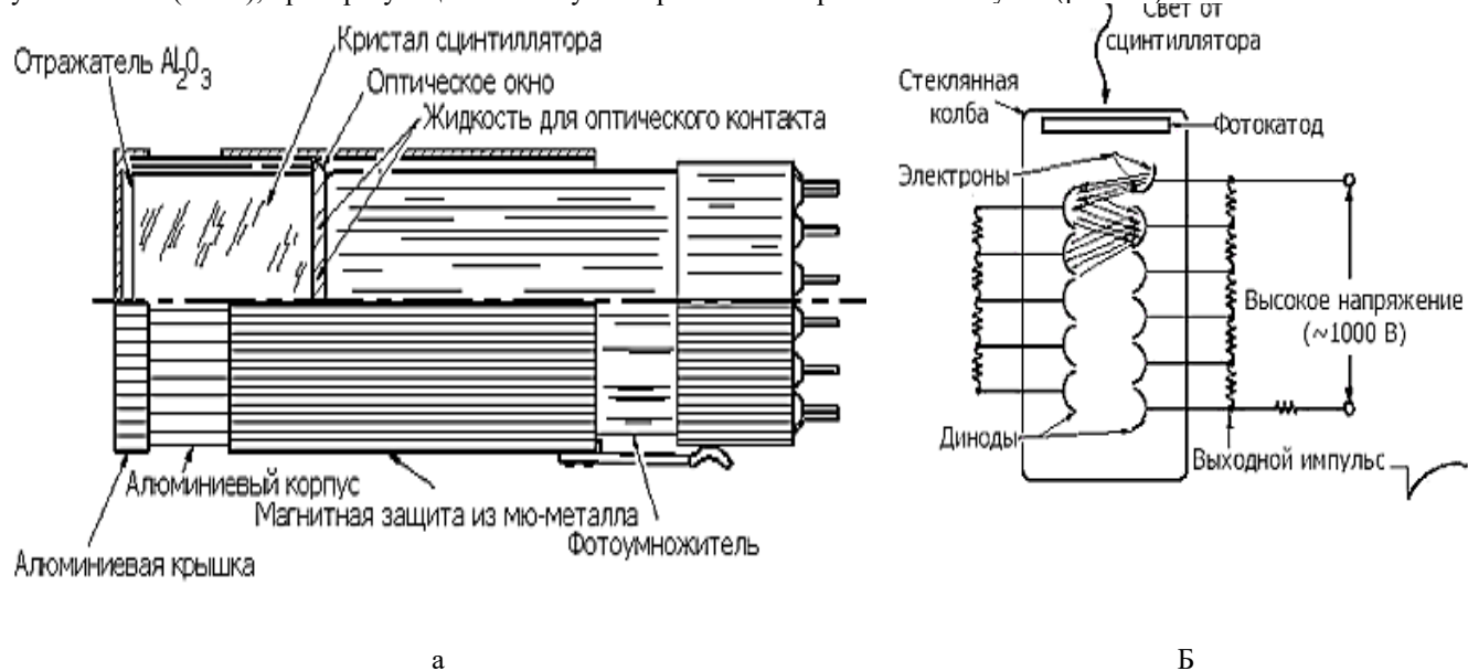
Рисунок 2.6 – Сцинтилляционный детектор: а) сцинтиллятор и ФЭУ; б) устройство ФЭУ
