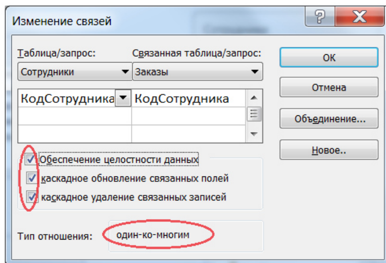
Рисунок 6 – Настройка связи между таблицами
