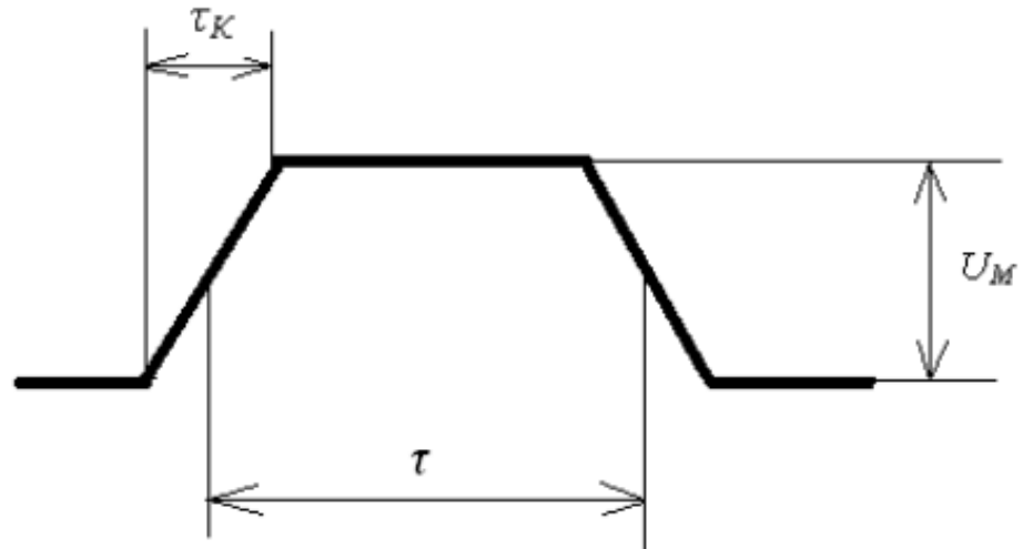
Рисунок 2- Трапецевидный импульс
