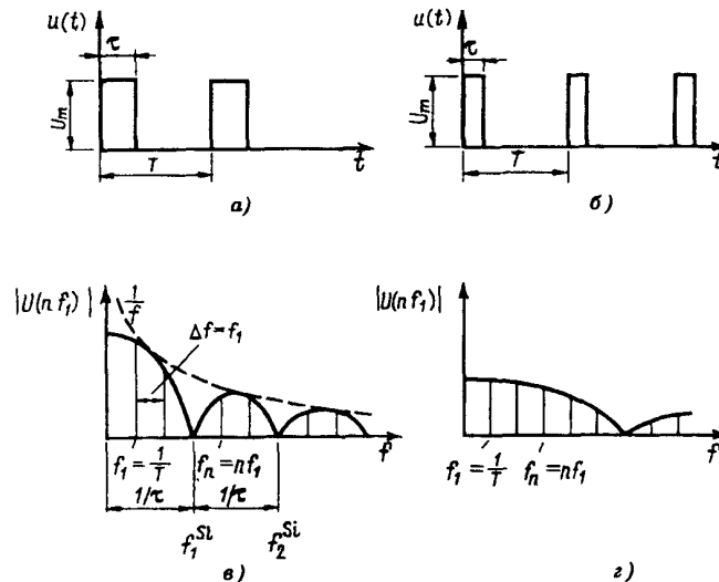
Рисунок 4 – Линейчатые спектры двух периодических последовательностей прямоугольных импульсов напряжений с личной скважностью (1:2): функция Si(x) - огибающая спектральных амплитуд (сплошная кривая); функция 1/f - огибающая функции Si(x) (пунктирная кривая)
