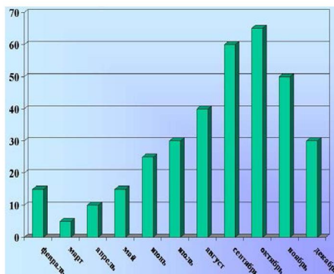
Рисунок 2. Годовое количество осадков
