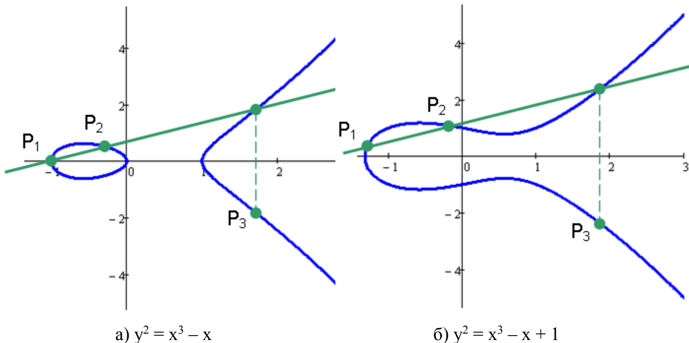
Рис.2. Сложение точек
