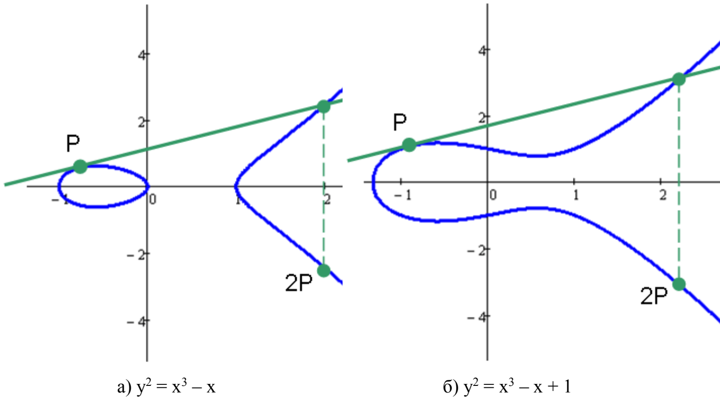
Рис.3. Удвоение точки
