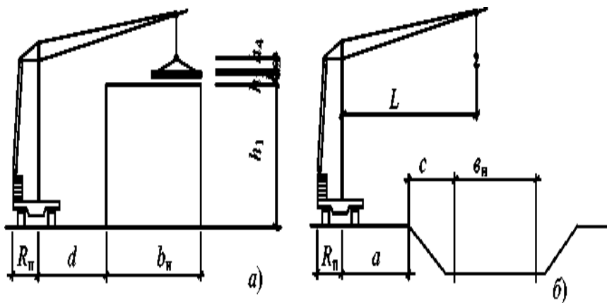
Рис. схемы определения необходимого вылета крюка башенного крана: при возведении надземной (а) и подземной (б) части здания
