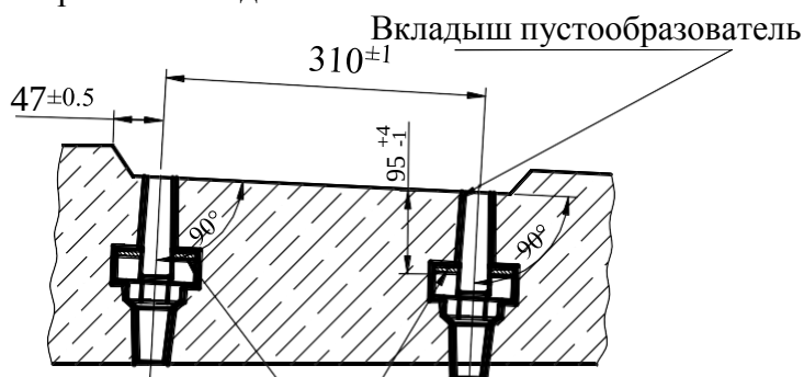
Рис. 7.3. Нормативная геометрическая модель подрельсовой части шпалы.
