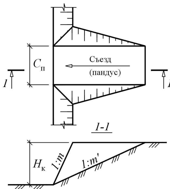
Рис.7. Схема въездной траншеи (пандуса)
