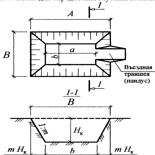
Рис.4. Схема для определения глубины котлована
