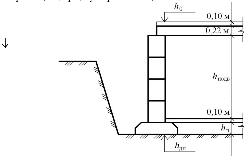
Рис.4. Схема для определения глубины котлована
