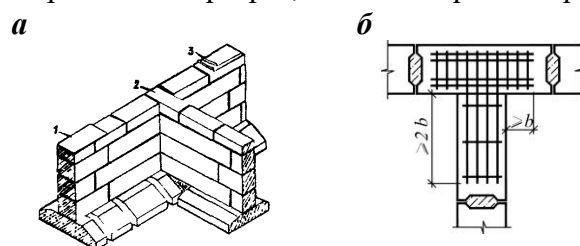
Рис. 2. Перевязка блоков продольных и поперечных стен подвала: а – перевязка блоков; б – усиление примыкания арматурными сетками; 1 – выровненная поверхность стены подвала; 2 – перевязка блоков; 3 – гидроизоляция.
