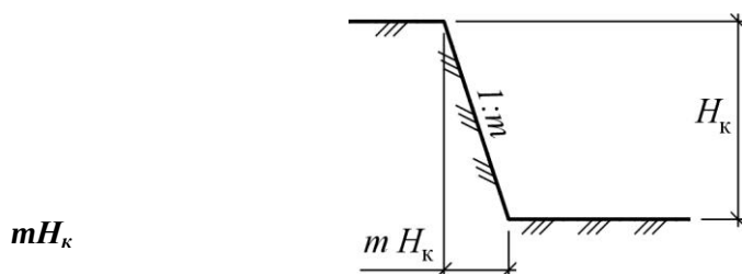
Рис. 3. Схема откоса
