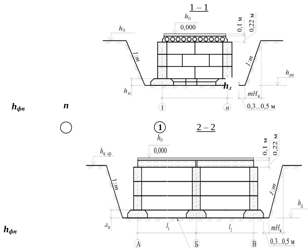
Рис. 1. Окончание 1-1 – продольный разрез; 2-2 – поперечный разрез
