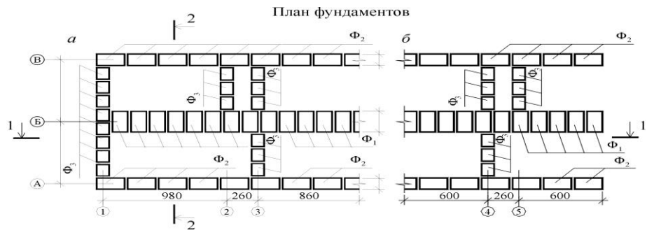
Рис. 1. Планы фундаментов и раскладки плит перекрытия над подвалом: a – для торцевой блок-секции; б – для рядовой блок-секции
