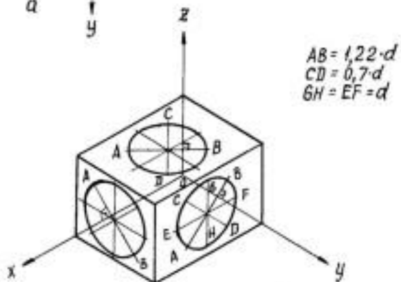
Прямоугольная изометрия
