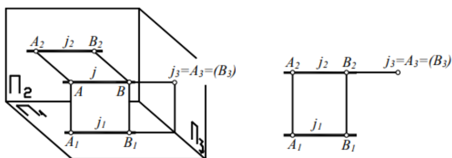
Рис.13. Профильно-проецирующая прямая
