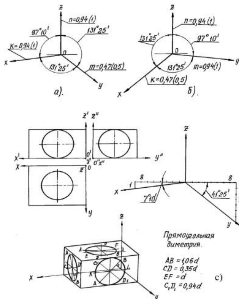
Прямоугольная диметрия
