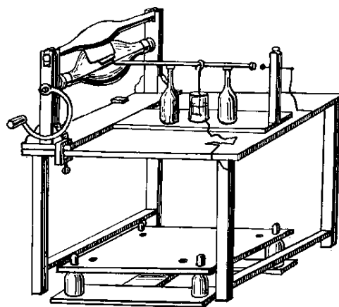
Рисунок 6. Электростатическая машина Болотова
