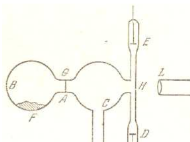
Рис.1 Опыт Содди
