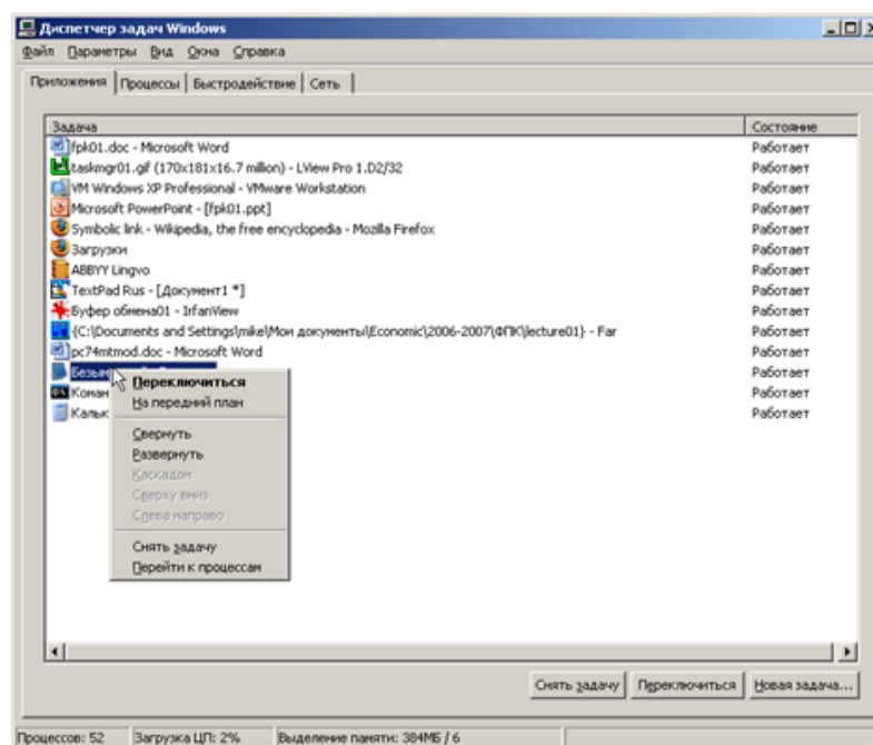
Рис. 13. Приложение Блокнот
