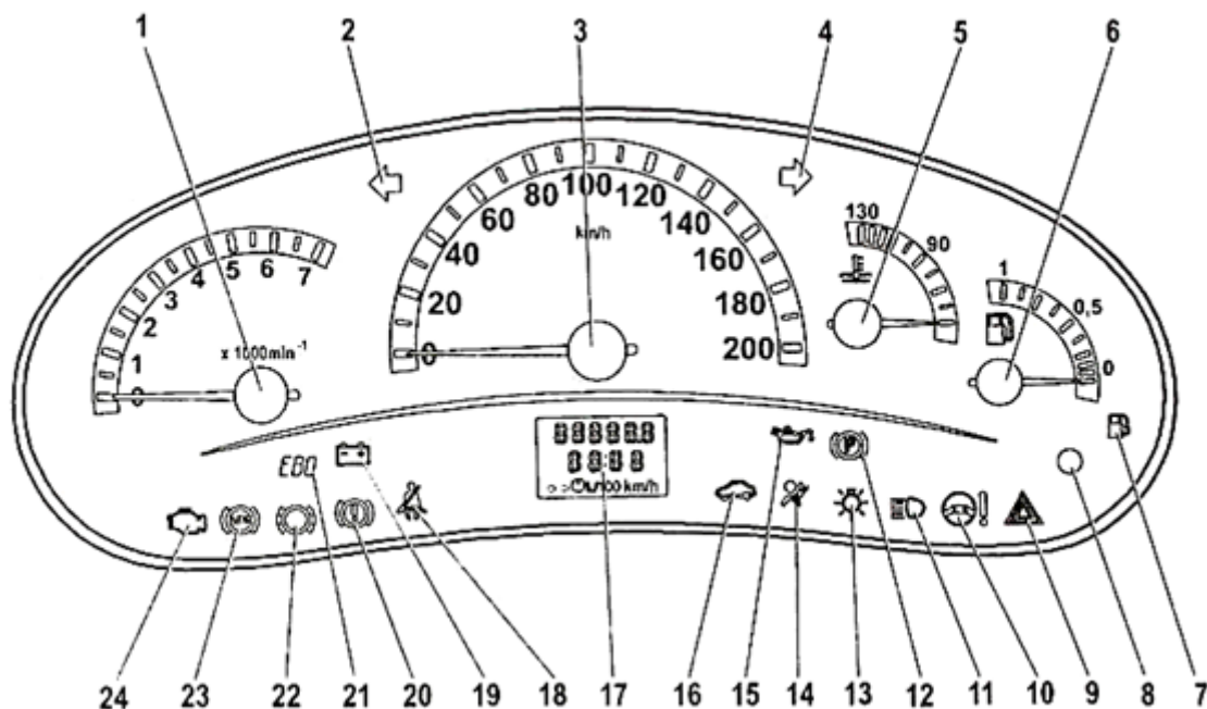
Рисунок2-ПриборнаяпанельавтомобиляЛады-Приоры (ВАЗ-2170):
