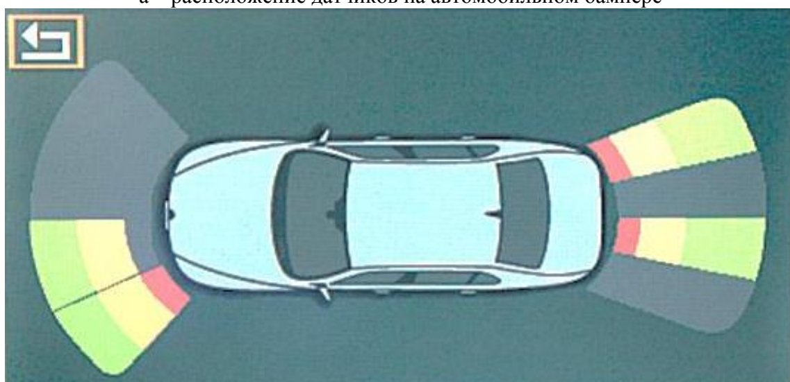
б – цветное отображение расстояния на дисплее до препятствия
