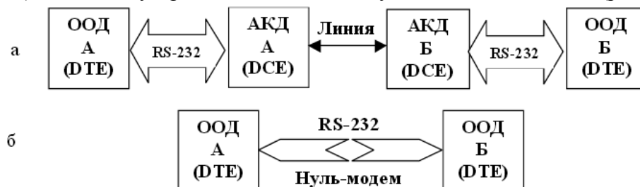
Рис. 17. Полная схема соединения:
