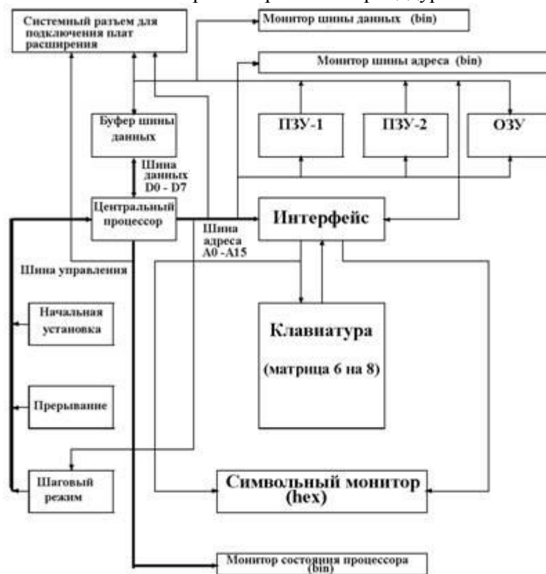
Рис. 1 Структурная схема центрального блока УМК
