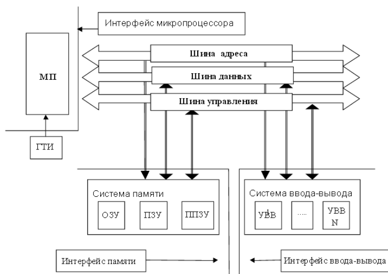
Рис. 1. Обобщенная структура МПС
