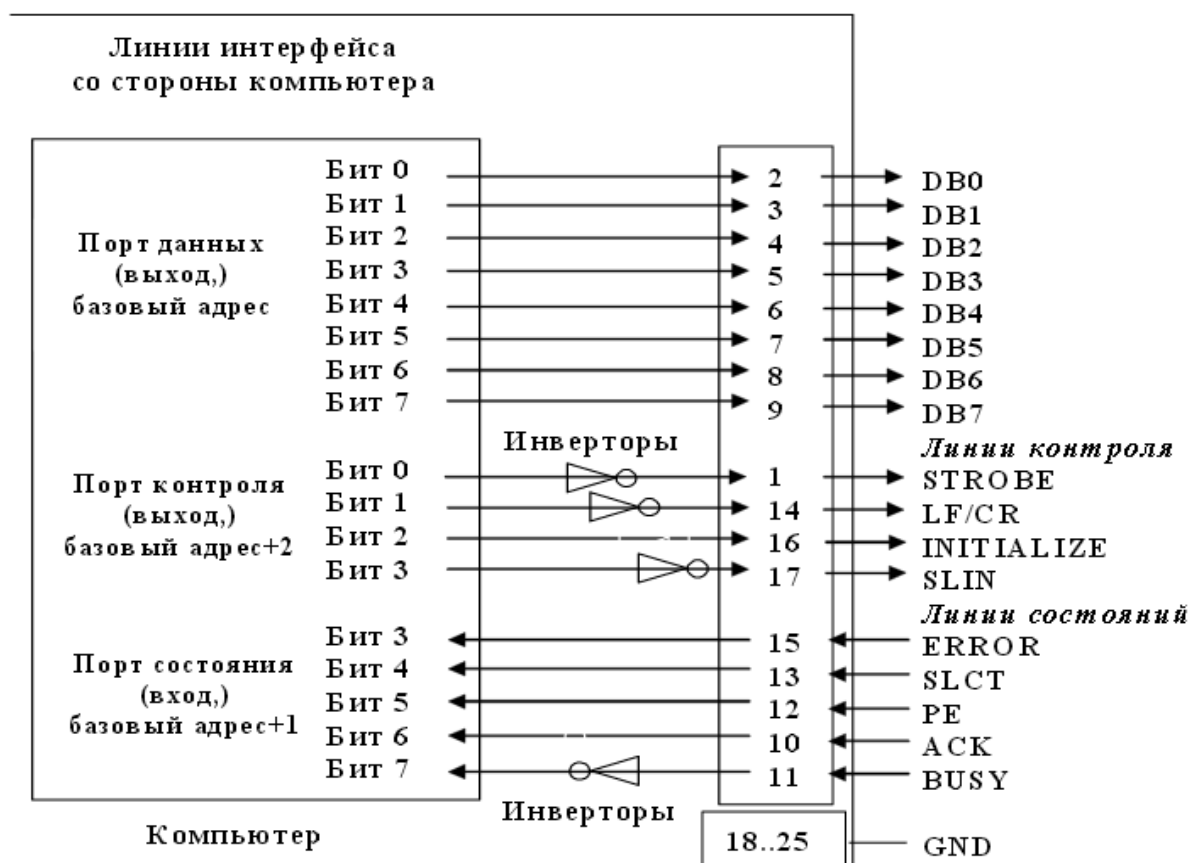
Рис. 12. Логическая структура параллельного порта
