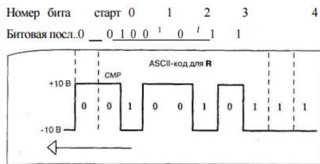
Рисунок 1.-Сигнал стандартаRS232при передаче символа «R».
