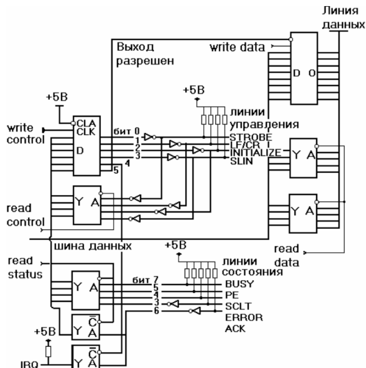
Рис. 11. Общая схема параллельного порта
