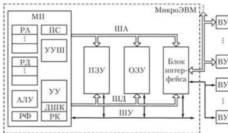
Рис. 1. Структура микропроцессорной системы
