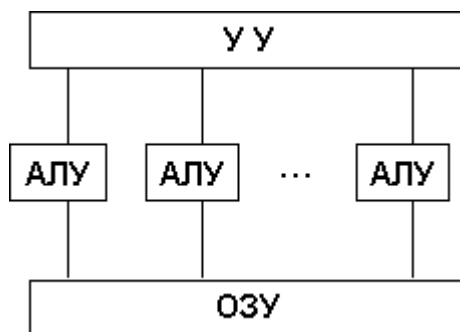
Рис. 2.4. Архитектура с параллельным процессором
