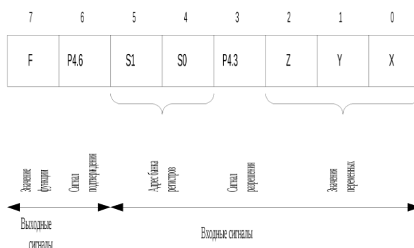
Рис. 26.14. Распределение разрядов порта P4 между входными и выходными сигналами
