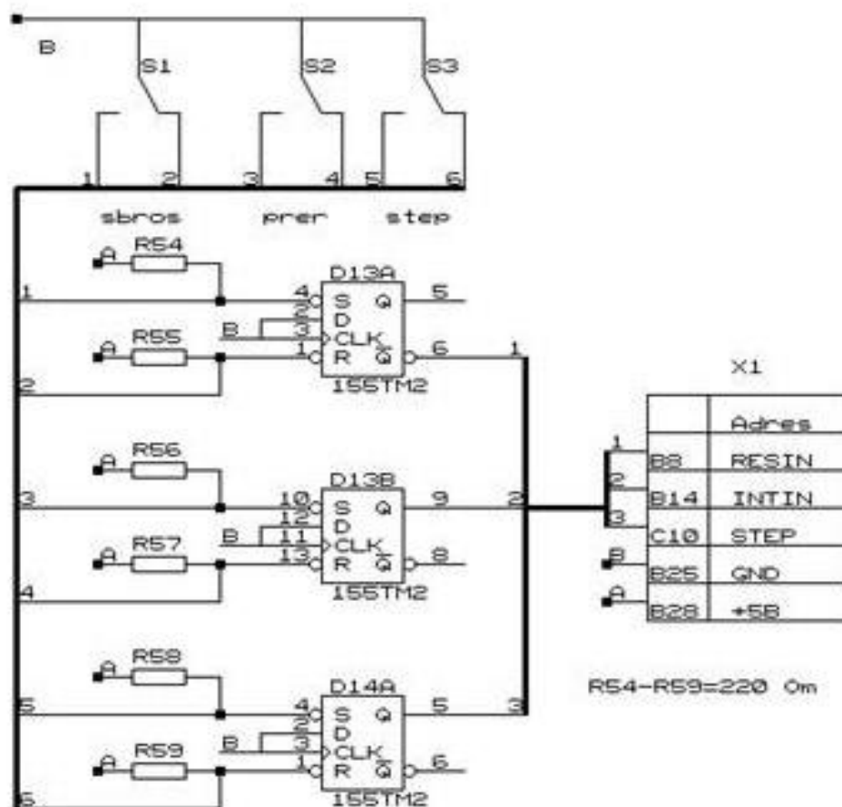
Рис. 3 Схема формирования сигнала "STEP" и устранения дребезга контактов аппаратными средствами
