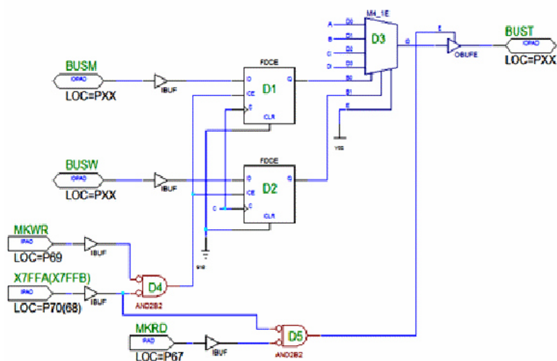
Рис. 29.8. Вариант подключения четырёх источников через мультиплексор (управление от регистра адреса)
