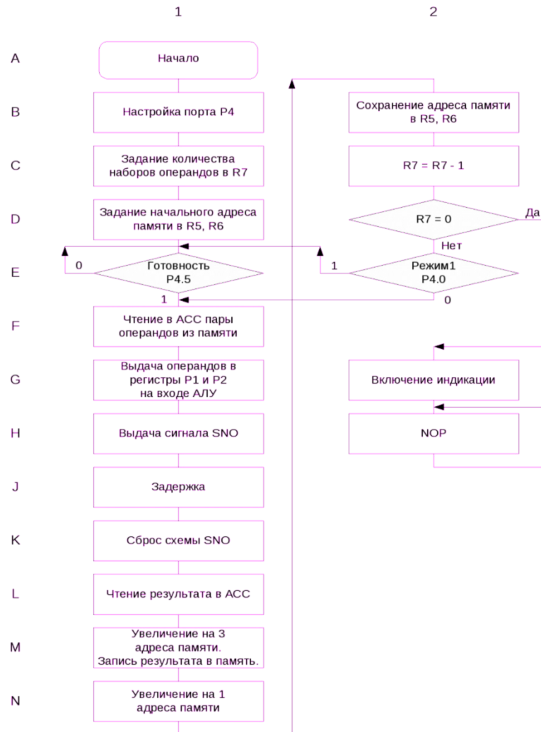
Рис. 28.4. Блок-схема программы
