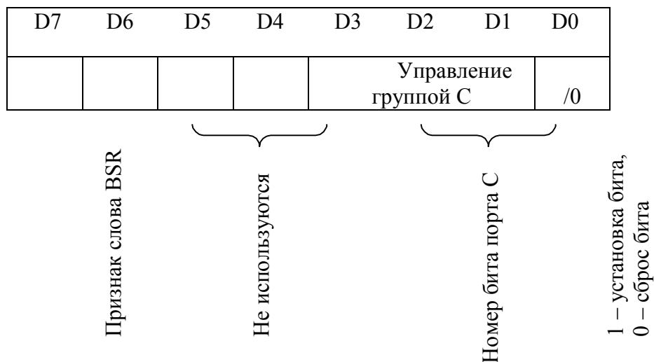
Рис. 3. Формат регистра BSR
