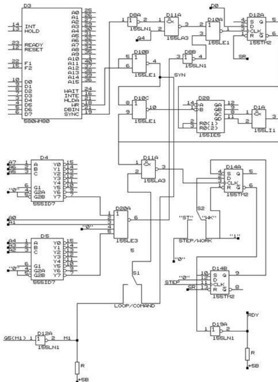
Рис. 4 Схема порта шагового режима
