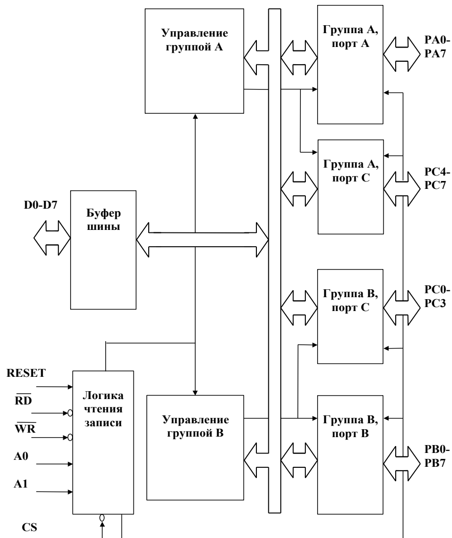
Рис. 1. Структурная схема БИС ППА К580BV55А
