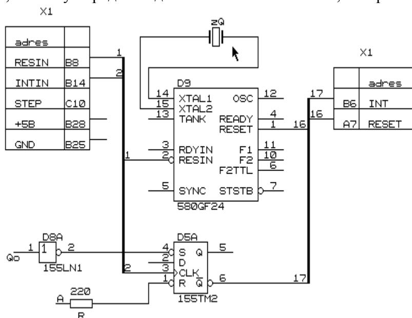
Рис. 2 Схема формирования сигнала “RESET”
