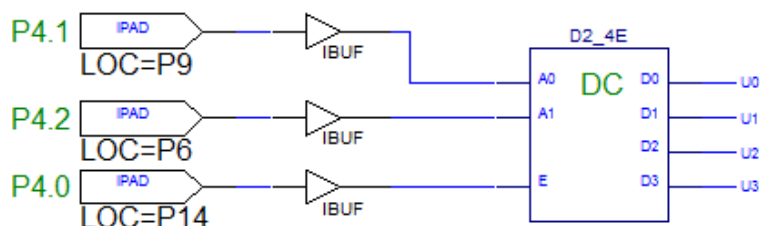
Рис. 29.14. Схема ввода в порт P4 нескольких битовых сигналов
