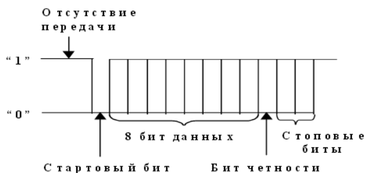
Рис. 14. Формат данных RS-232C
