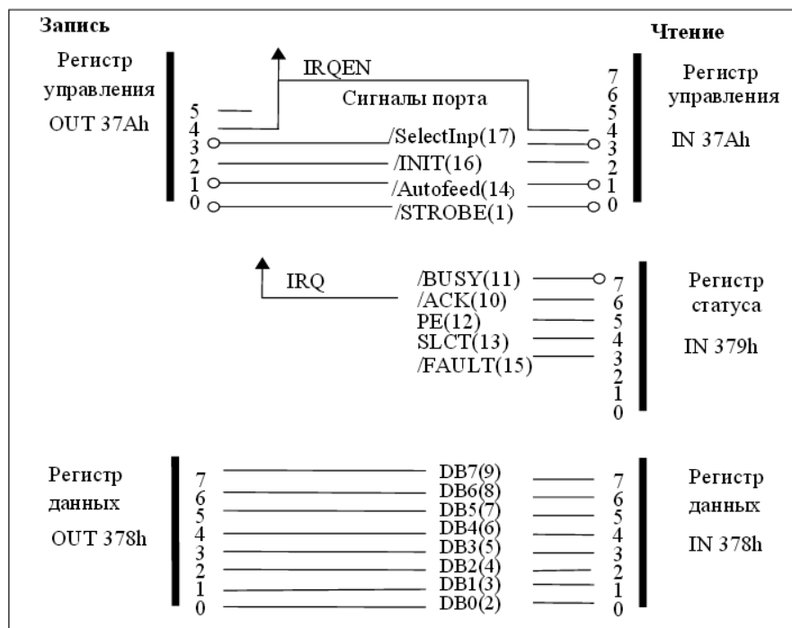
Рис. 10. Сигнал интерфейса Centronics
