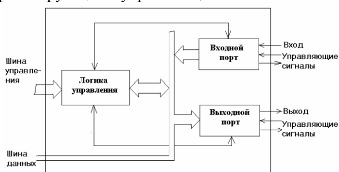
Рис. 2. Интерфейс, обеспечивающий последовательную связь между двумя системами.
