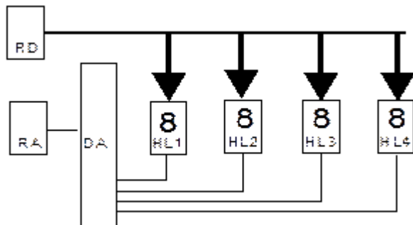
Структурная схема динамической индикации
