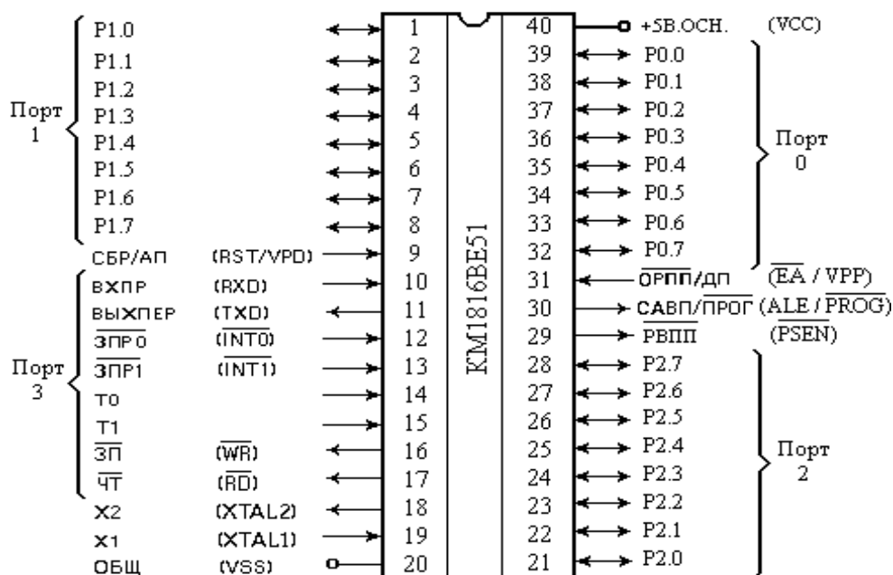
Рис. 3.1. Цоколёвка корпуса МК51 и наименование выводов
