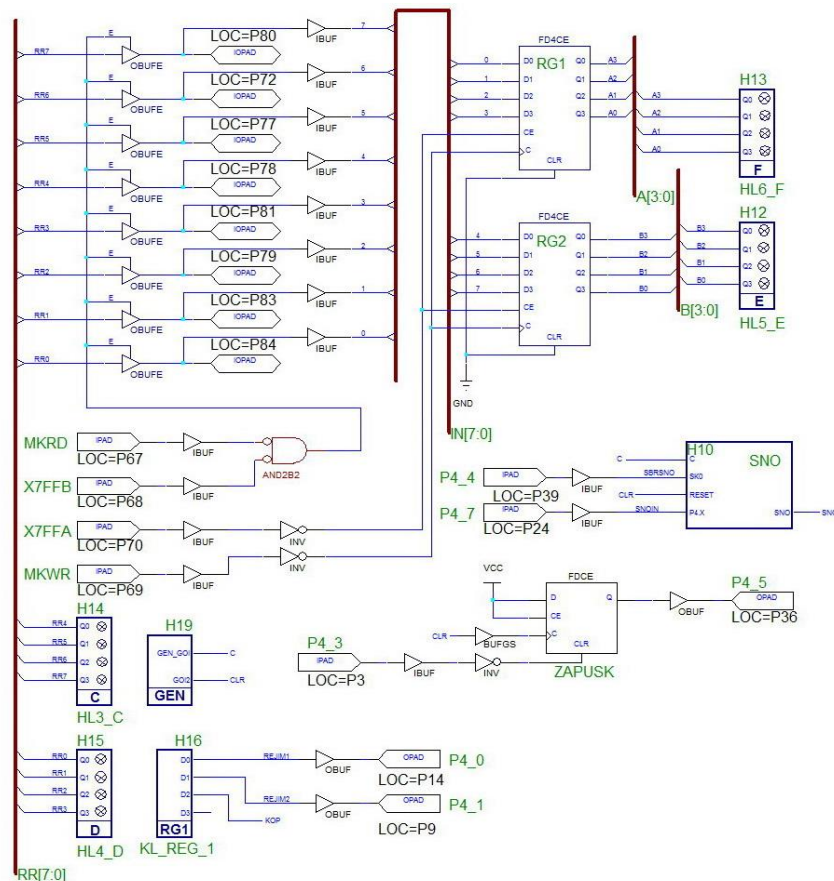
Рис .28.3. Схема подключения АЛУ к МК
