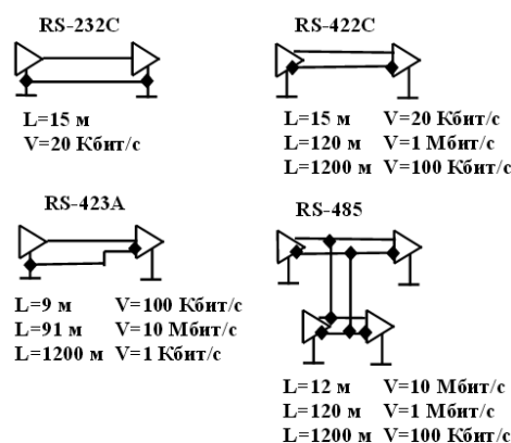
Рис. 16. Стандарты последовательного интерфейса
