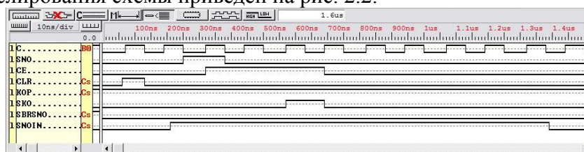
Рис. 28.1. Схема привязки сигнала SNO к тактовым сигналам
