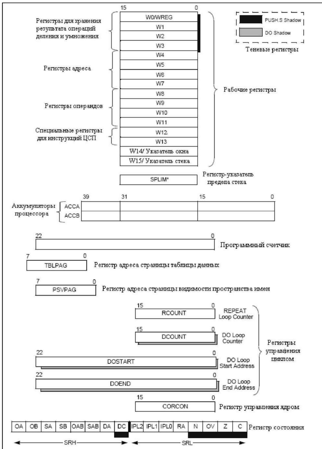
Рисунок 8 - Регистры микропроцессора
