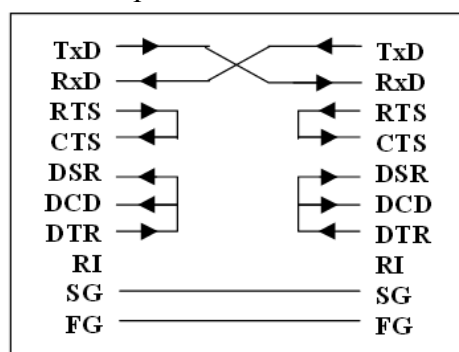
Рис. 13. Схема 4-проводной линии связи для RS-232C
