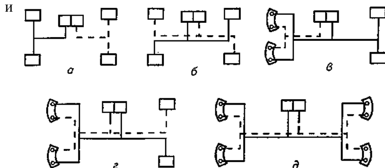
Рис. 7. Схема двухконтурных тормозных приводов: а — по осям; б—диагональная; в — с дублированием передних тормозов; г — с дублированием передних тормозов и раздельным управлением каждого заднего; д — с полным дублированием
