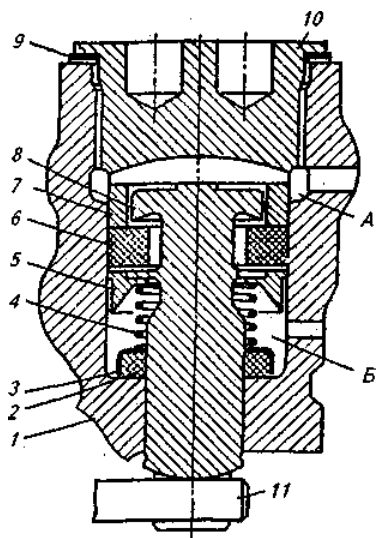
Рис. 21. Регулятор давления автомобиля ВАЗ-2121: А, Б- полости регулятора; 1 — корпус; 2—уплотнительное кольцо; 3—обойма; 4—пружина; 5—тарелка; 6 — резиновый уплотнитель; 7-распорная втулка; 8— поршень; 9—прокладка; 10— пробка; 11 — торсион привода регулятора
