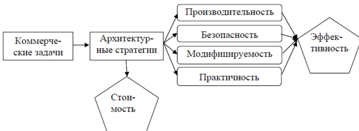
Рисунок 4.4 - Контекст метода анализа стоимости и эффективности (СВАМ)
