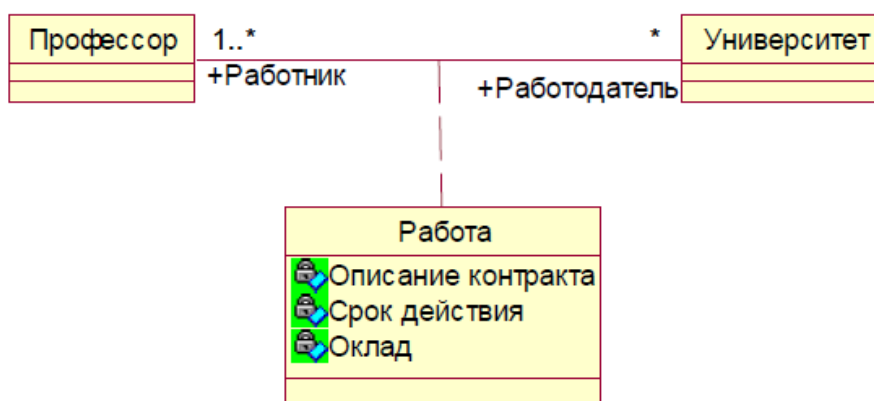
Рисунок 1.6 - Структура объектно-ориентированной программы в виде связанных классов
