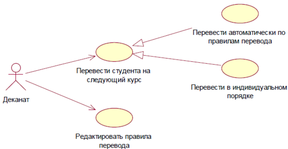
Рисунок 3.7 - Диаграмма вариантов использования «Перевод, отчисление, ликвидация задолженностей»
