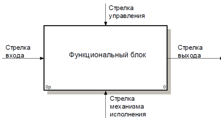
Рисунок 2.19 - Соединение стрелок со сторонами функционального блока
