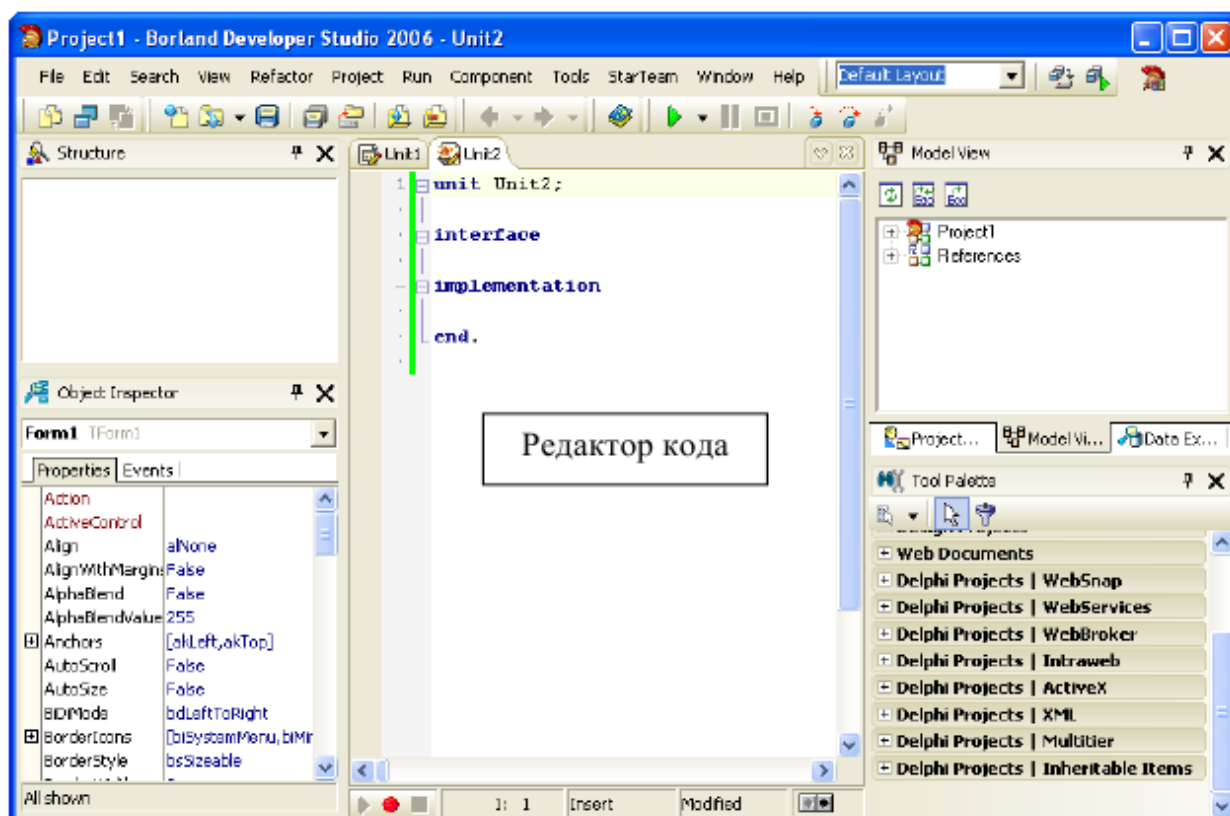
Рисунок 5.5 - Новый модуль
