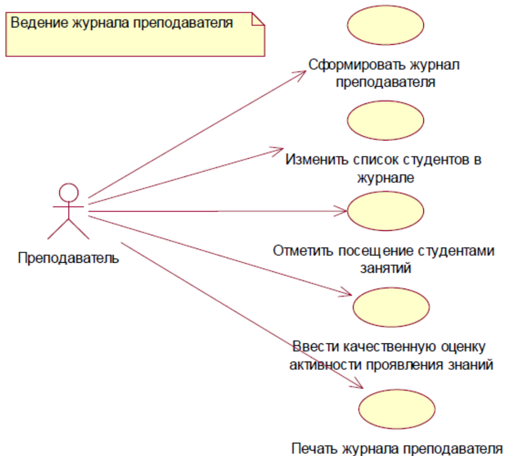
Рисунок 3.5 - Диаграмма вариантов использования «Ведение журнала преподавателя»
