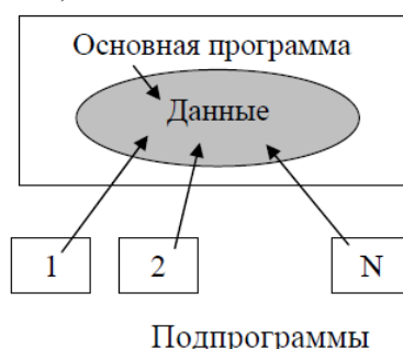
Рисунок 1.3 - Принцип работы программ с глобальной областью данных
