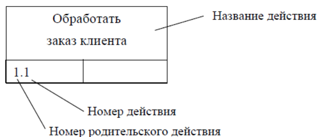
Рисунок 2.8 - Изображение и нумерация действия в диаграмме IDEF3
