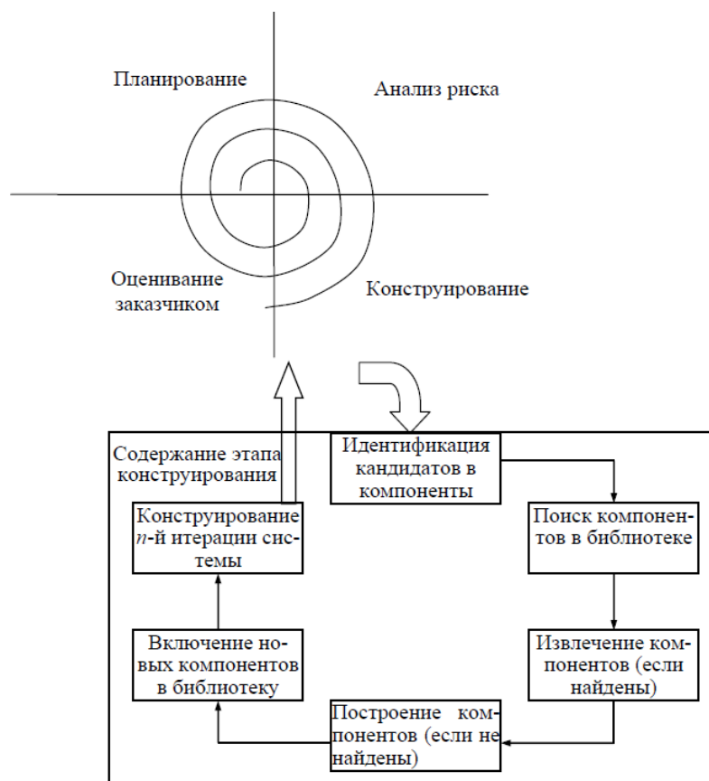
Рисунок 1.15 - Компонентно-ориентированная модель
