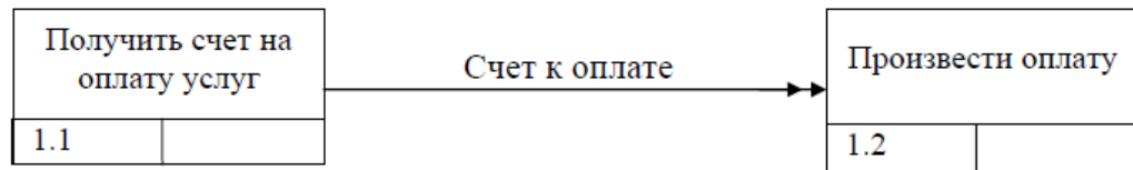
Рисунок 2.10 - Объектная связь между действиями 1.1 и 1.2
