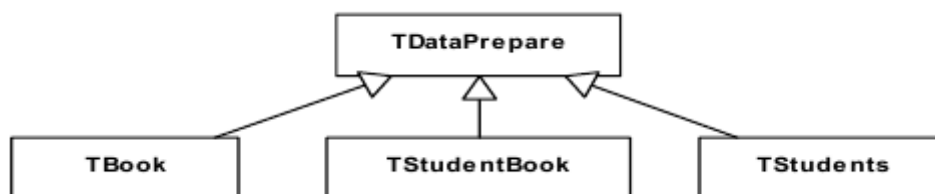
Рис. 5.7. Структура классов слоя «Бизнес-логика»
