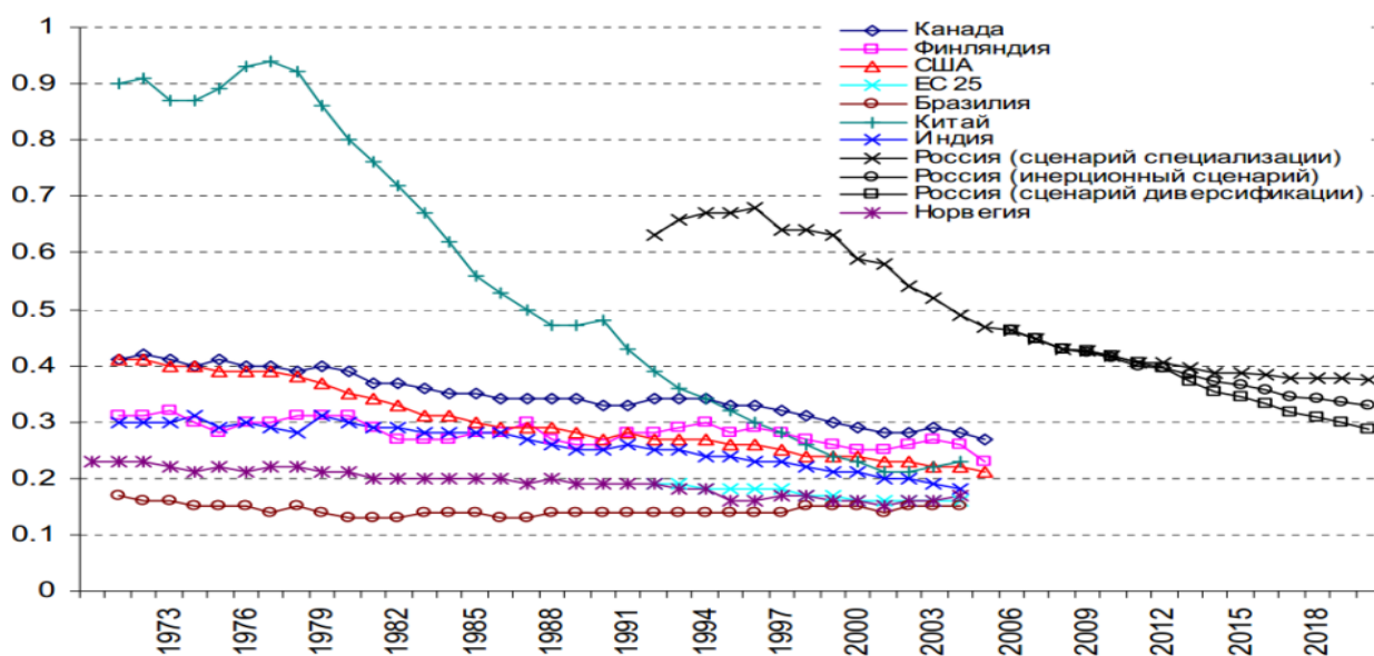
Рисунок.3.2 - Динамика энергоёмкости в ряде стран мира и России за период 1973-2018 гг. 3
