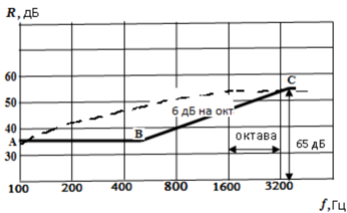
Рисунок 2 - Нормативная и расчетная характеристики звукоизоляции
