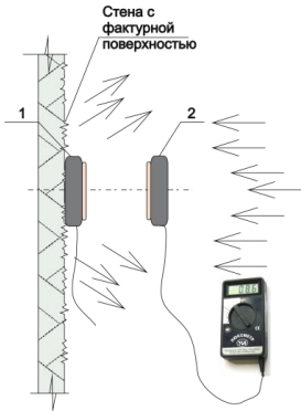
Рисунок 3.1 — Пример проведения замеров отраженного света люксметром (положения фотоэлемента при измерении светотражения различных по фактуре поверхностей стен): 1 — измерение падающего на поверхность стены света; 2 — измерение света, отраженного от поверхности стены Таблица 3.2 — Величина коэффициента светотражения
