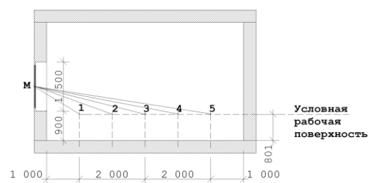
Рисунок 2.1 — Пример выполнения схем плана ( A ) и поперечного разреза ( Б ) помещения на прозрачной основе
