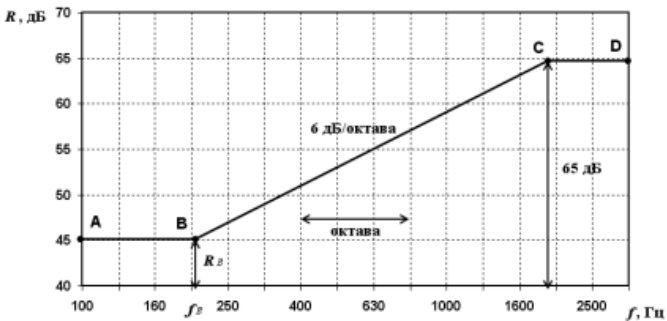
Рисунок 1 - Частотная характеристика звукоизоляции (шкала абсцисс – логарифмическая)
