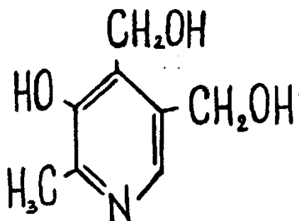
Пиридоксин
