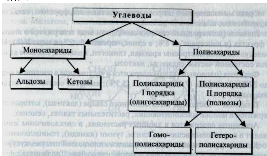
Рисунок 1. Классификация углеводов
