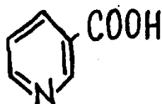
Никотиновая кислота
