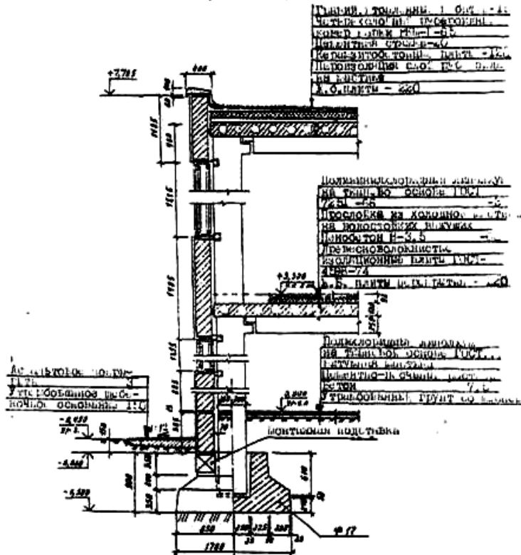
Разрез 3-3
