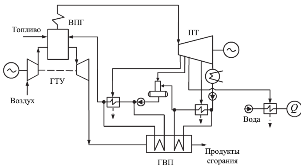
Рисунок 3.1 – Принципиальная тепловая схема ПГУ с ВПГ:
