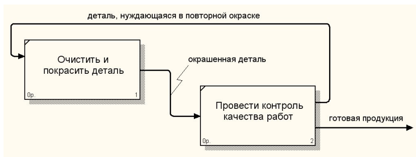
Рисунок 1.8 – Комбинированная стрелка выход – обратная связь на вход
