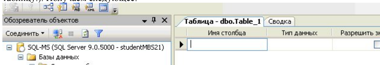
Рисунок 6. Создание таблицы
