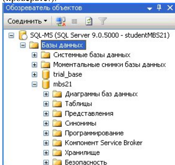
Рисунок 5. Обозреватель объектов
