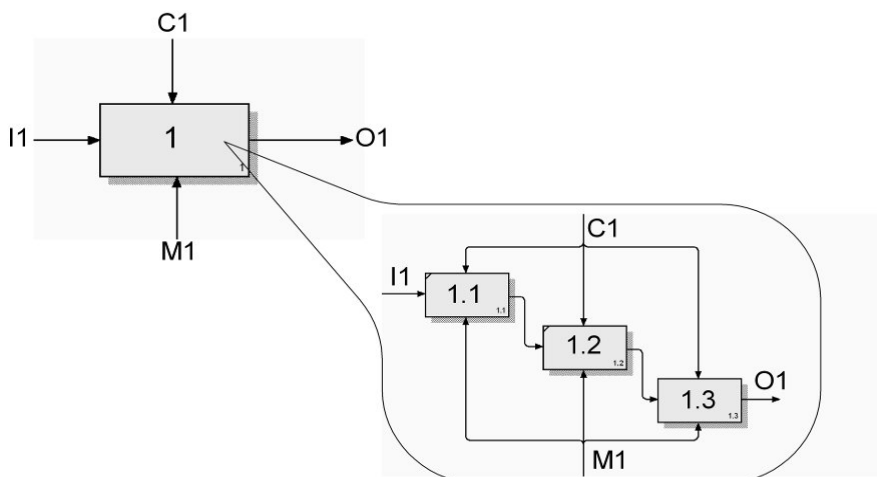
Рисунок 1.2 – Принцип декомпозиции
