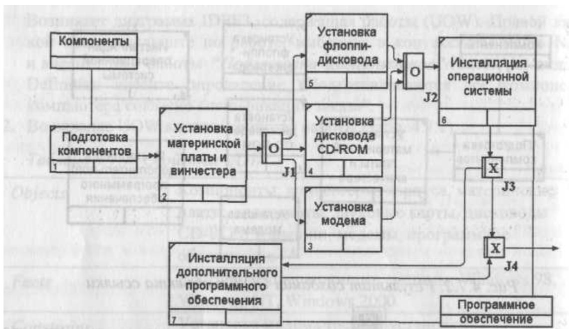
Рис. 4. Результат создания диаграммы IDEF3
