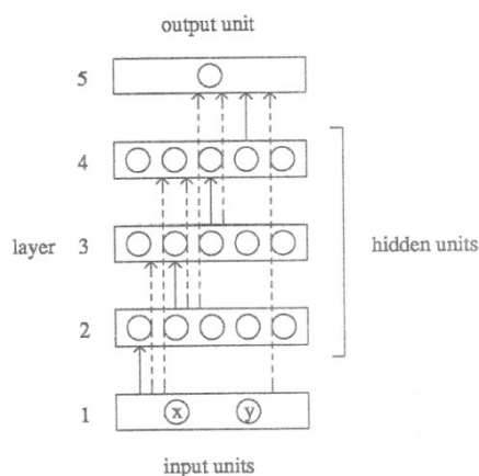
Рисунок 5.22 – Сверху структура предлагаемой сети в Matlab, снизу она же в виде обобщённой схемы
