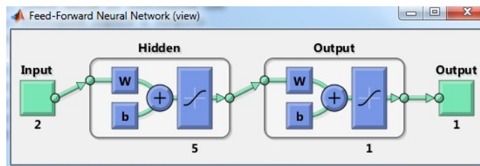
Рисунок 3.29 – Данная сеть тоже справится с задачей XOR
