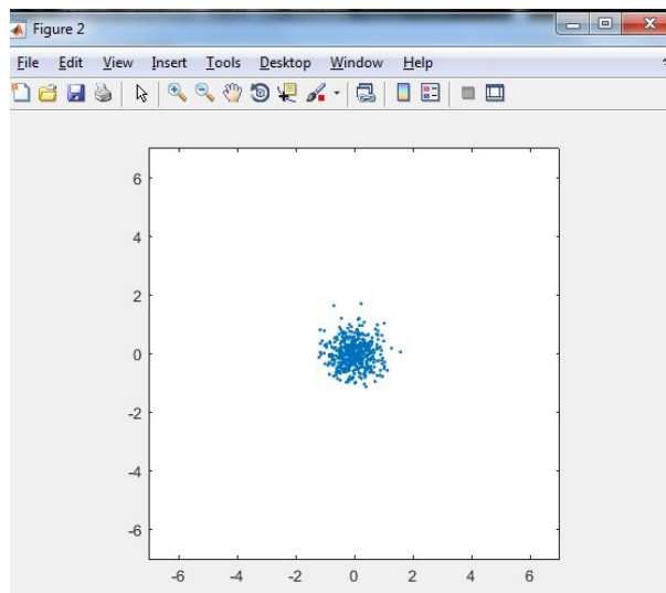
Рисунок 1.3 – Сгенерированное множество точек для случая \begin{matrix} \text{grid}^2 \\ 1 \end{matrix} \times \begin{matrix} \text{grid}^2 \\ 2 \end{matrix} \times 0.2, \begin{matrix} \text{grid}^2 \\ 12 \end{matrix} \times 0
