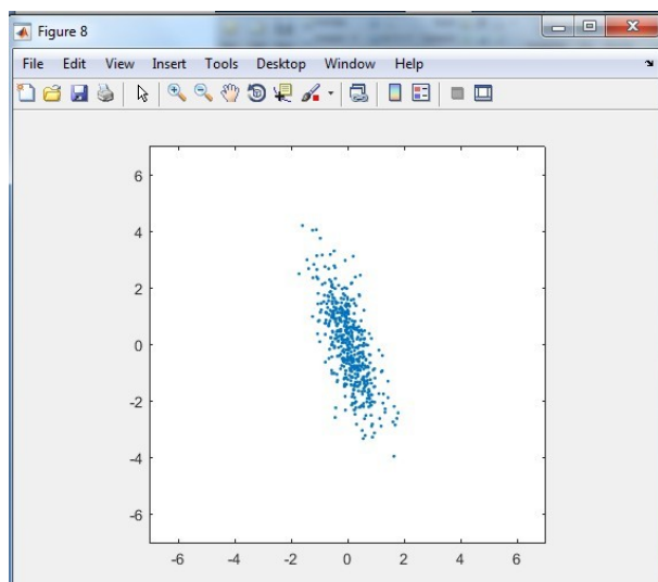
Рисунок 1.9 – Сгенерированное множество точек для случая \xi_1^4 \propto 0.3 , \xi_2^2 \propto 2 , \xi_{12} \propto 0.5
