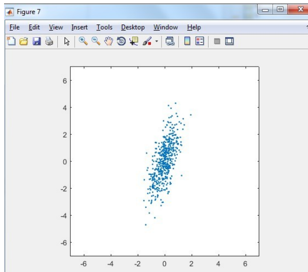
Рисунок 1.8 – Сгенерированное множество точек для случая \xi_1^2 \propto 0.3 , \xi_2^2 \propto 2 , \xi_{12} \propto 0.5
