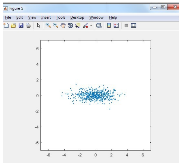
Рисунок 1.6 – Сгенерированное множество точек для случая \begin{matrix} \text{grid}^2 \\ 1 \end{matrix} \propto 2, \begin{matrix} \text{grid}^2 \\ 2 \end{matrix} \propto 0.2, \begin{matrix} \text{grid} \\ 12 \end{matrix} \propto 0
