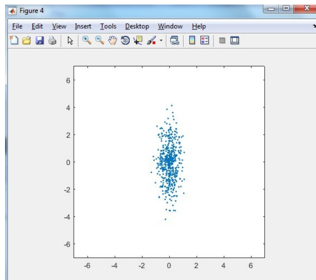
Рисунок 1.5 – Сгенерированное множество точек для случая \begin{matrix} \text{grid}^2 \\ 1 \end{matrix} \propto 0.2, \begin{matrix} \text{grid}^2 \\ 2 \end{matrix} \propto 2, \begin{matrix} \text{grid} \\ 12 \end{matrix} \propto 0
