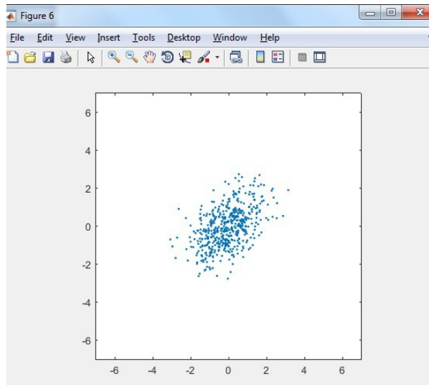
Рисунок 1.7 – Сгенерированное множество точек для случая \xi_1^2 \propto \xi_2^2 \propto 1 , \xi \propto 0.5
