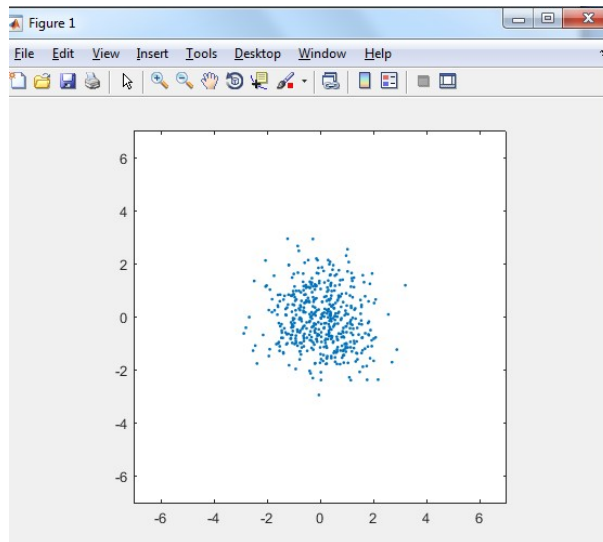
Рисунок 1.2 – Сгенерированное множество точек для случая \begin{matrix} \text{grid}^2 \\ 1 \end{matrix} \times \begin{matrix} \text{grid}^2 \\ 2 \end{matrix} \times \begin{matrix} \text{grid}^2 \\ 12 \end{matrix} \times 0
