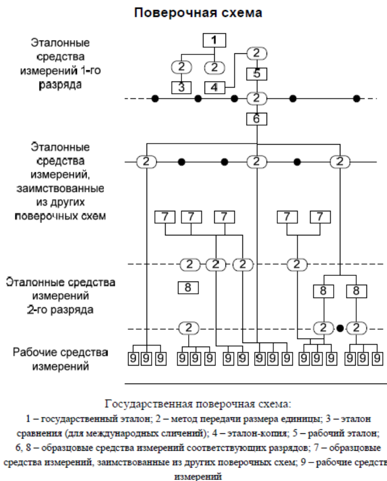
Рис. 2. Пример поверочной схемы.
