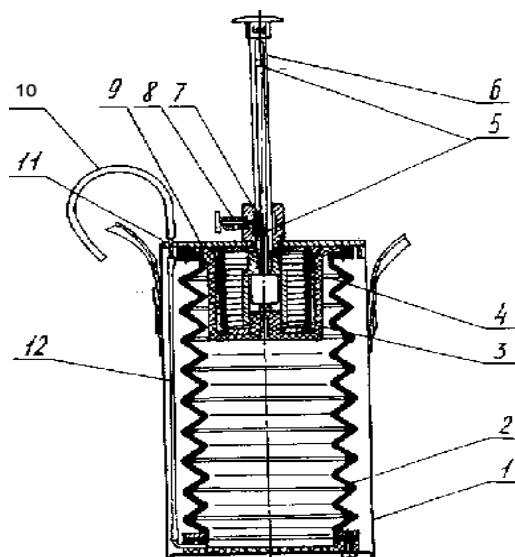
Рисунок 3.1 – Устройство газоанализатора УГ-2: 1 – корпус, 2 – сильфон, 3 – пружина, 4 – кольцо распорное, 5 – канавка с двумя углублениями, 6 – шток, 7 – втулка, 8 – фиксатор, 9 – плата, 10 – трубка резиновая, 11 – штуцер, 12 – трубка резиновая
