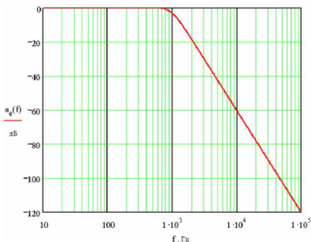
Рисунок 1 - АЧХ фильтра
