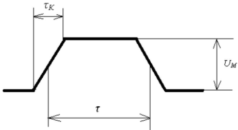
Рисунок 2- Трапециевидный импульс
