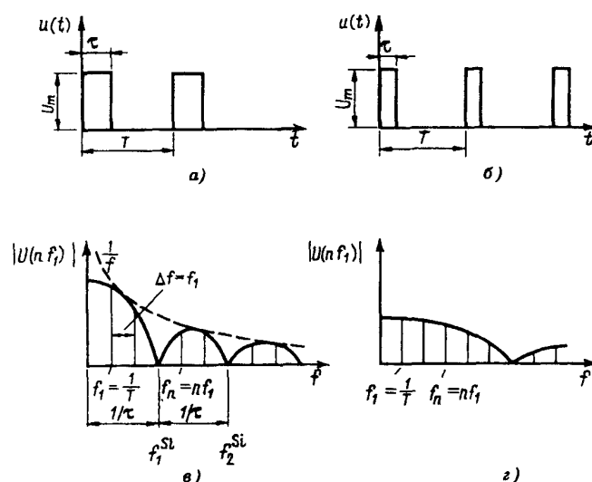
Рисунок 4 – Линейчатые спектры двух периодических последовательностей прямоугольных импульсов напряжений с различной скважностью (1:2): функция Si(x) – огибающая спектральных амплитуд
