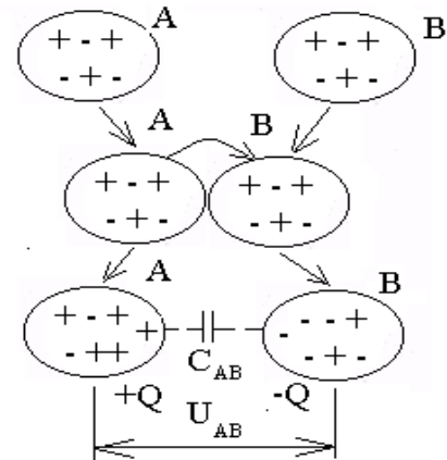
Рисунок 2. Электризация за счет трения
