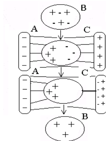
Рисунок . 1 Электризация за счет индукции
