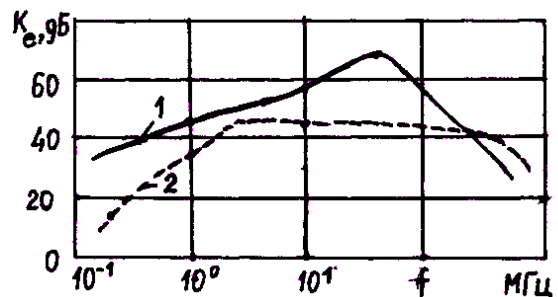
Рисунок 4 - Пример сетевого фильтра на 220 В, ток 1 А, а) схема, б) частотные зависимости: 1 – противофазные помехи, 2 – синфазные помехи
