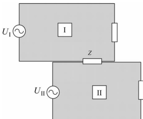
Рисунок 1 – Гальванический путь передачи ЭМС
