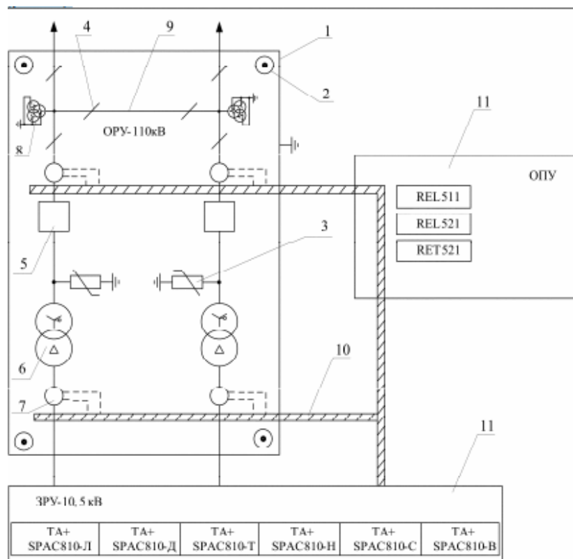
Рисунок 1 - Принципиальная схема расположения терминалов защиты 1 – контур заземления; 2 – молниеотвод; 3 – ОПН; 4 – разъединитель; 5 – выключатель; 6 – трансформатор; 7 – трансформатор тока; 8 – трансформатор напряжения; 9 – шина; 10 – кабельный лоток; 11 – общестанционный пункт управления
