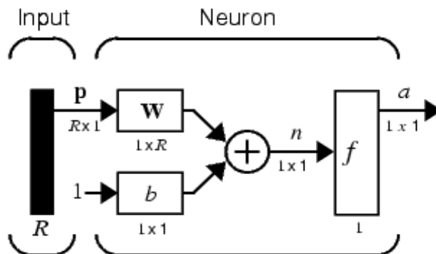
Рис. 6.3. Укрупненная схема нейрона с векторным входом
