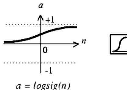
Рис. 6.6. Логистическая функция активации
