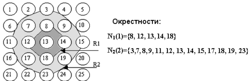
Рис. 12.3. Окрестности радиусов 1 и 2 нейрона-победителя с номером 13.
