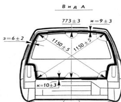
Рис.9.Размеры проемов и зазоры сопрягаемых деталей кузова автомобиля модели ВАЗ-1111
