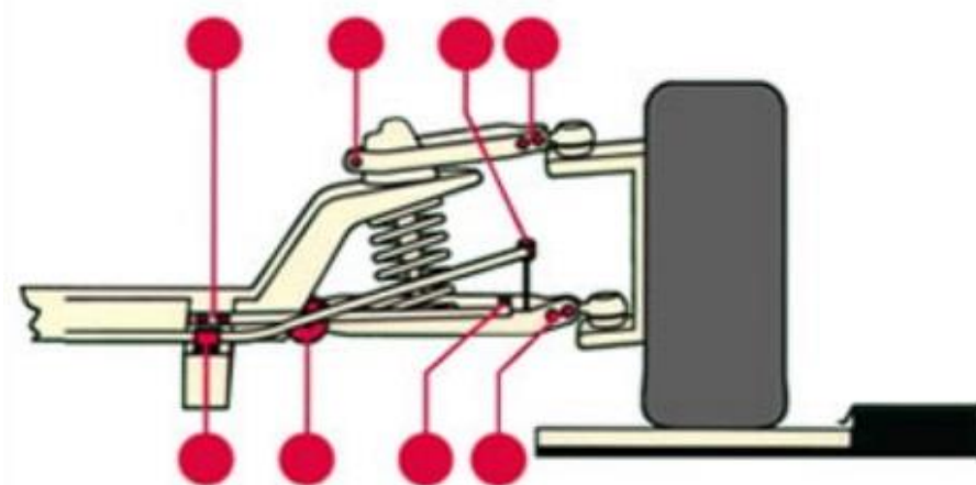
Рисунок 10. Точки контроля в подвеске автомобиля
