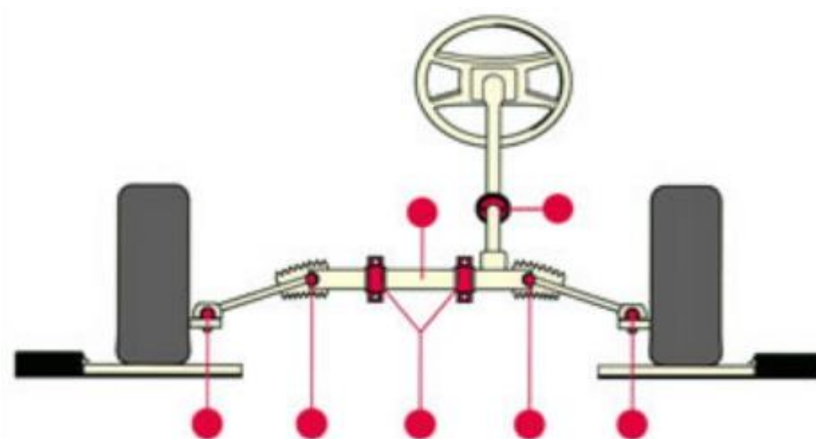
Рисунок 9. Точки контроля в рулевом механизме
