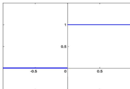
Рисунок 3.2 – График функции Хевисайда
