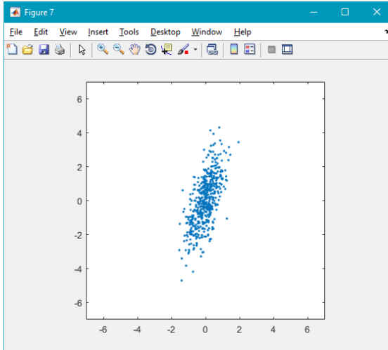
Рисунок 3.21– Сгенерированное множество точек для случая
