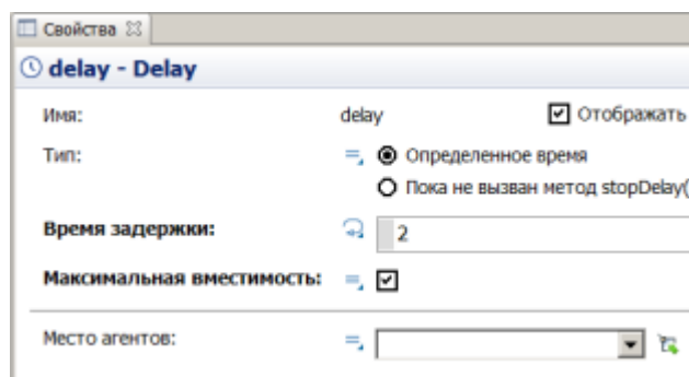
Рисунок 14.23 – Окно свойств объекта Delay
