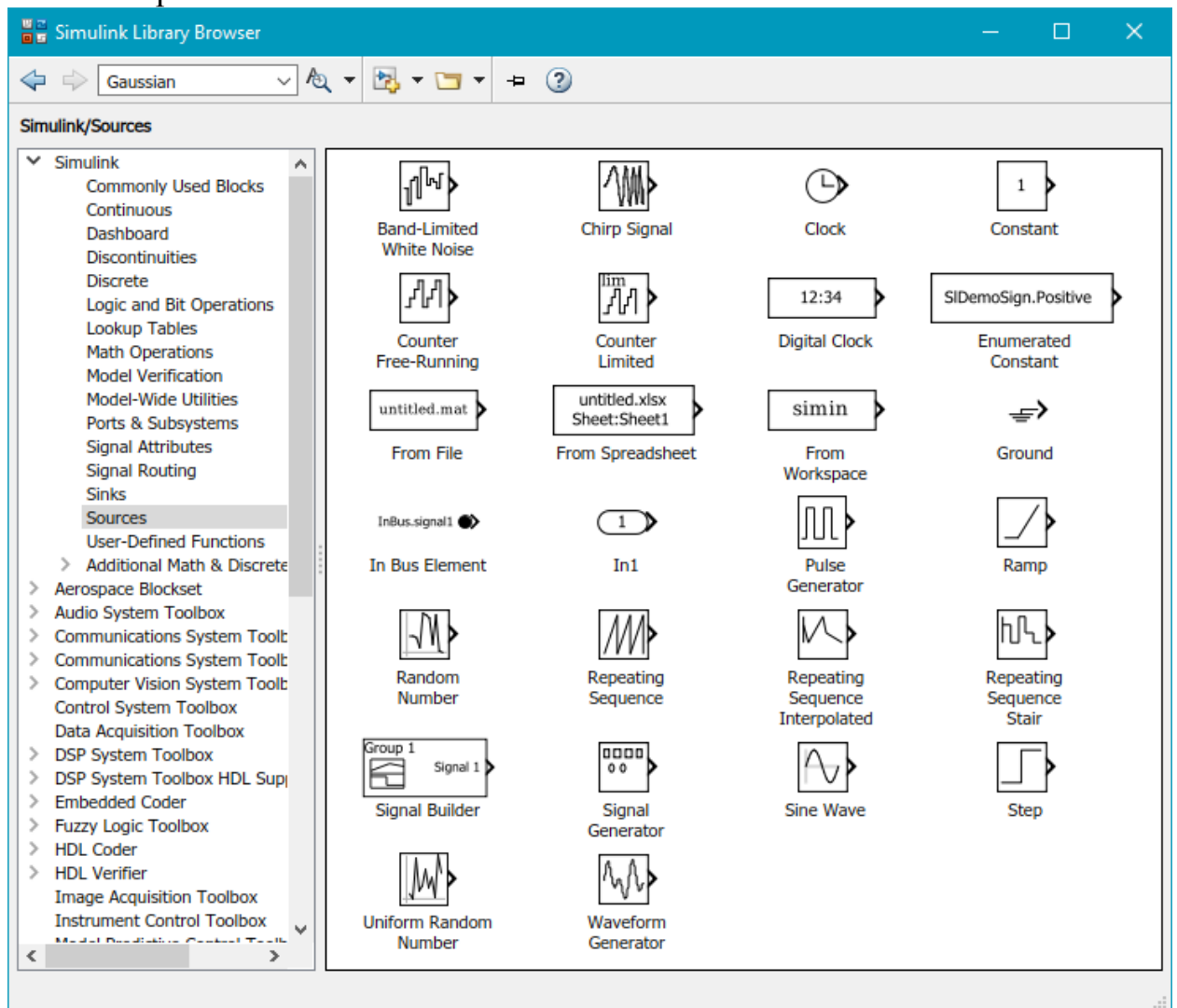
Рисунок 1.3 – Блоки библиотеки Simulink/Sources
