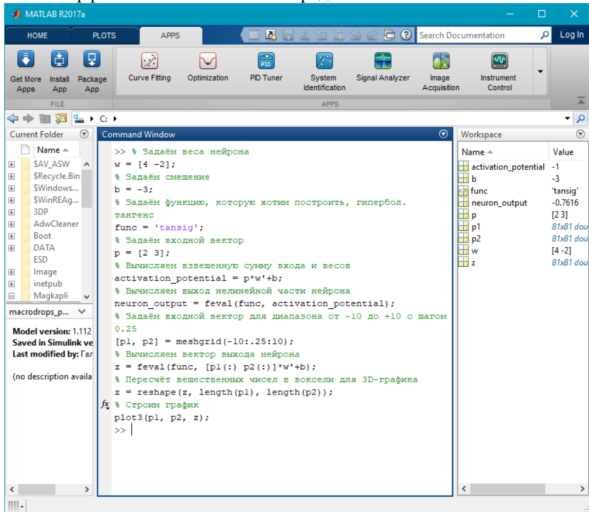
Рисунок 1.1 –Интерфейс системы MATLAB
