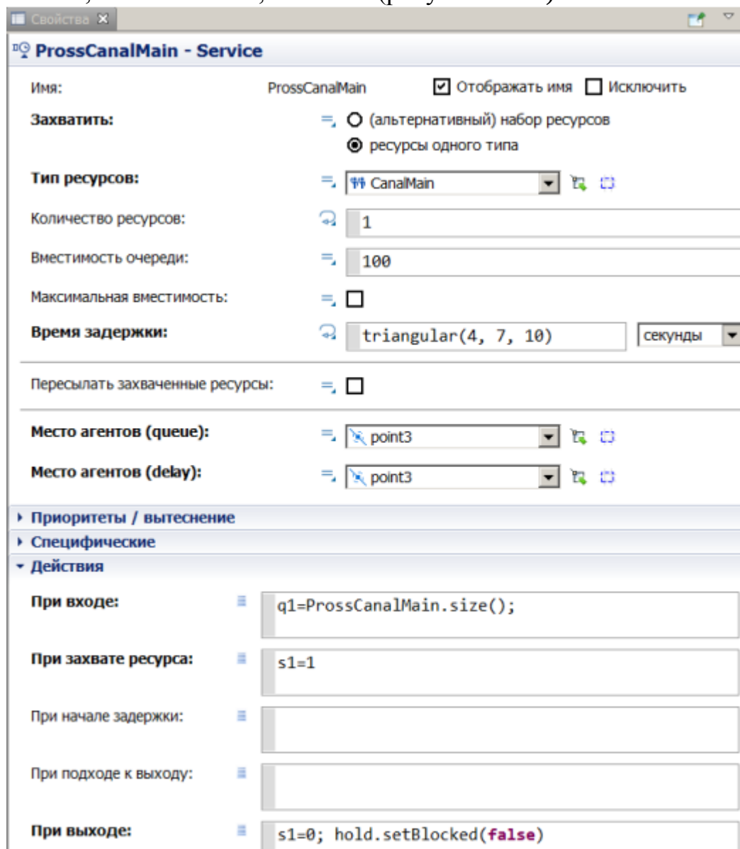
Рисунок 14.22– Окно свойств объекта ProssCanalMain
