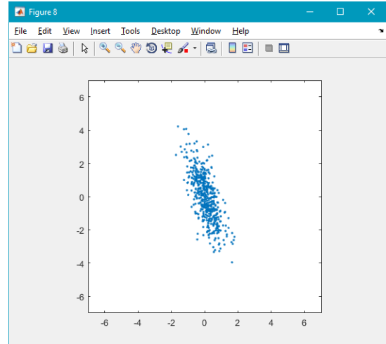
Рисунок 3.22– Сгенерированное множество точек для случая
