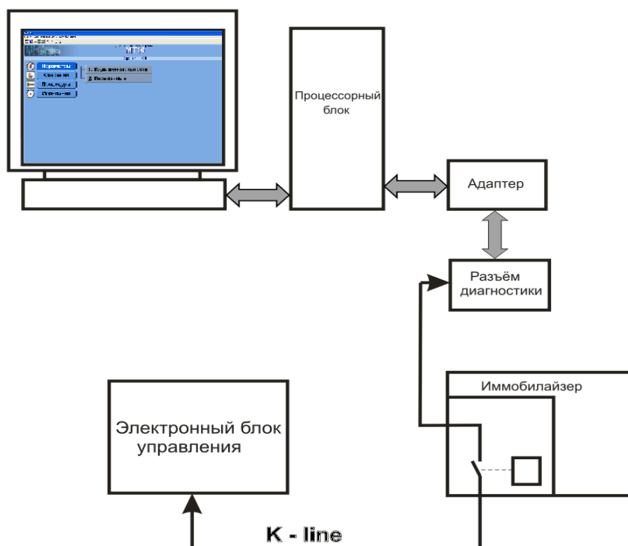
Рис. 12. Схема подключения диагностического сканера MT – 10.
