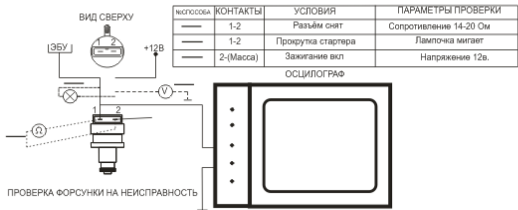
Рис. 20. Диагностика работы форсунки.
