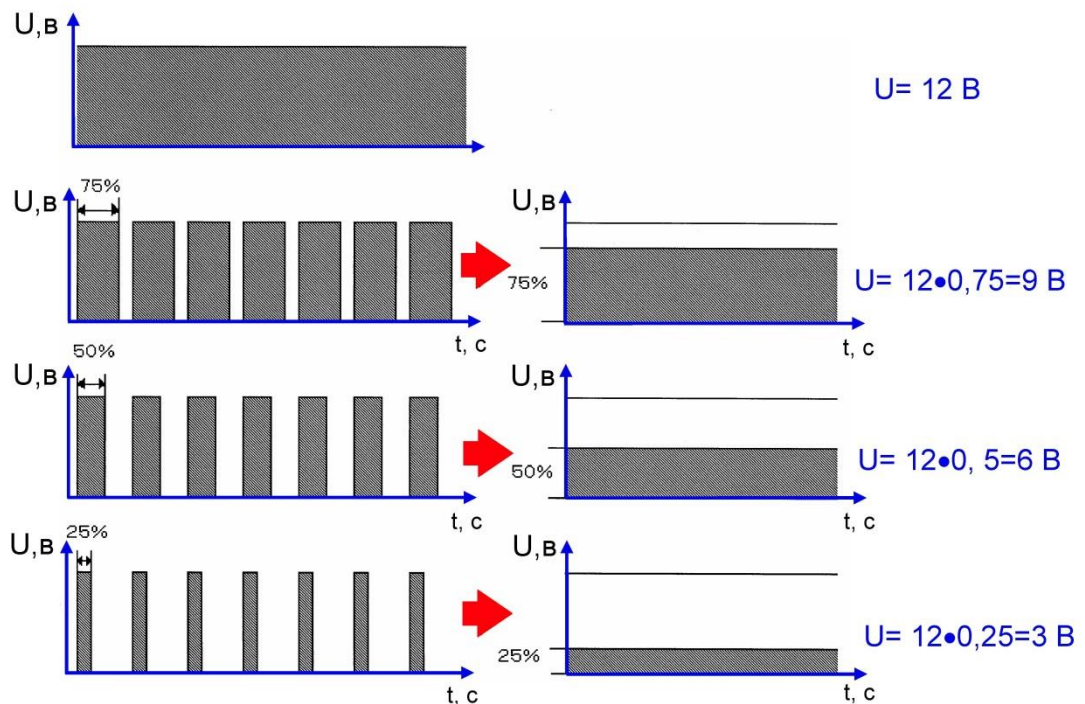
Рис. 1. Импульсный сигнал, отображаемый осциллографом и среднее напряжение выходного сигнала, измеряемое тестером.
