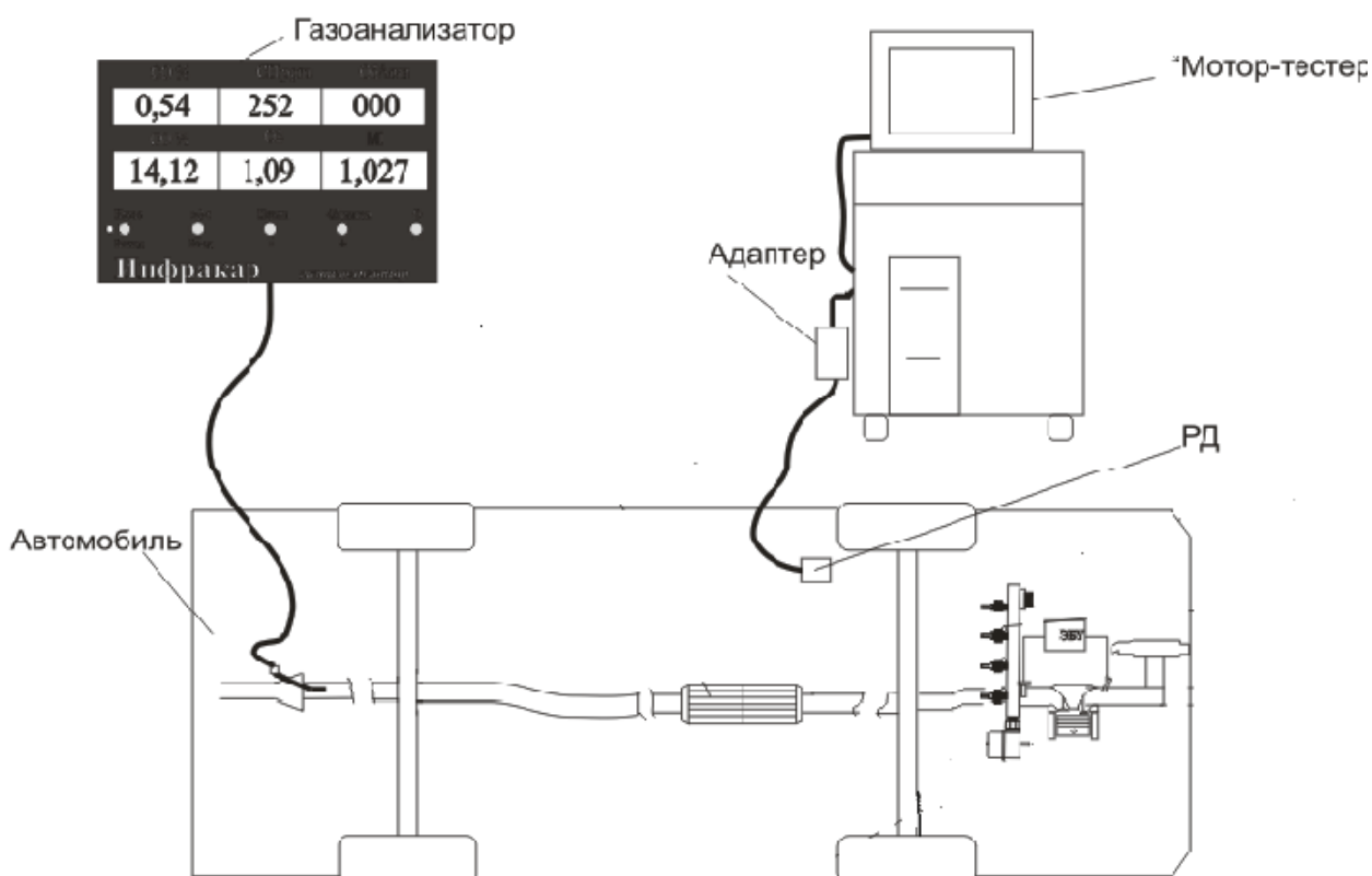
Рис. 12. Экспериментальная установка.
