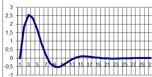
Переходный процесс 2
