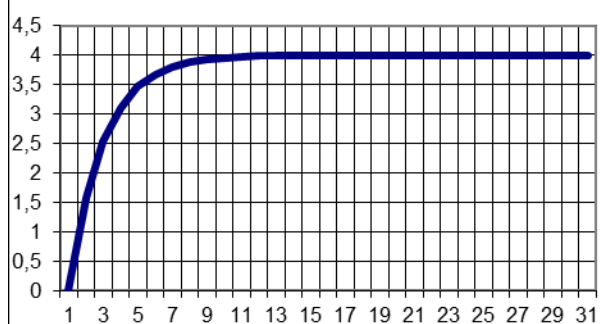
Переходный процесс 1
