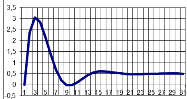
Переходный процесс 3
