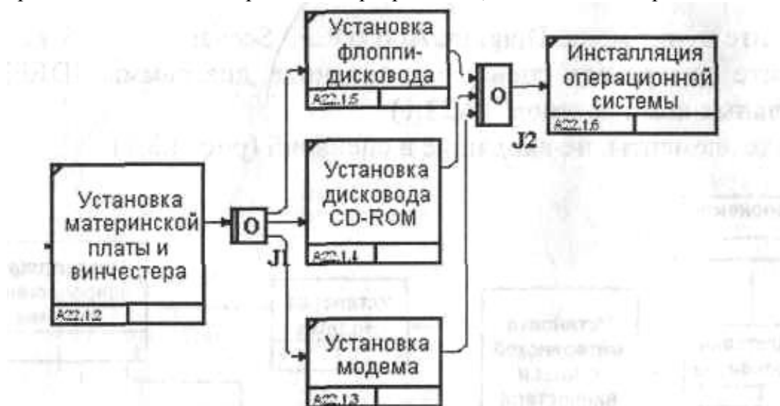
Рис. 3. Диаграмма IDEF3 после создания перекрестков
