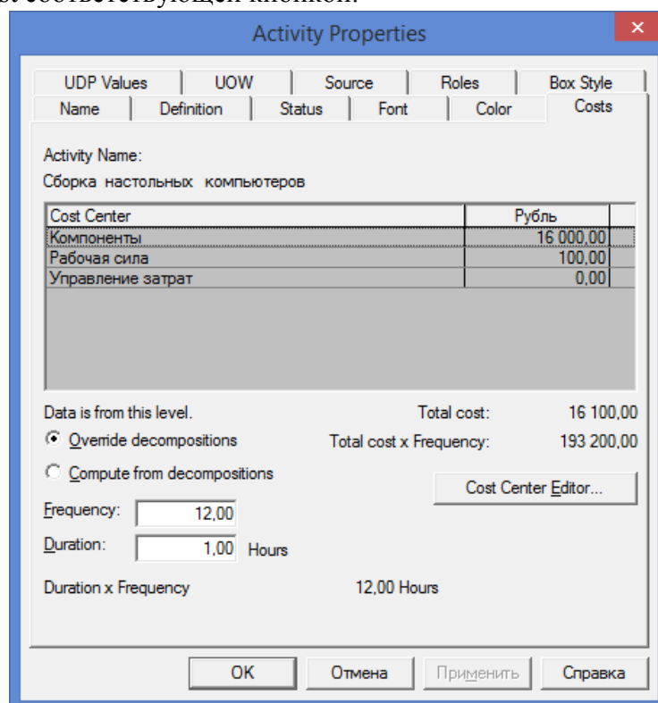
Рисунок 4 - Задание стоимости работ в диалоге Activity Properties/Cost
