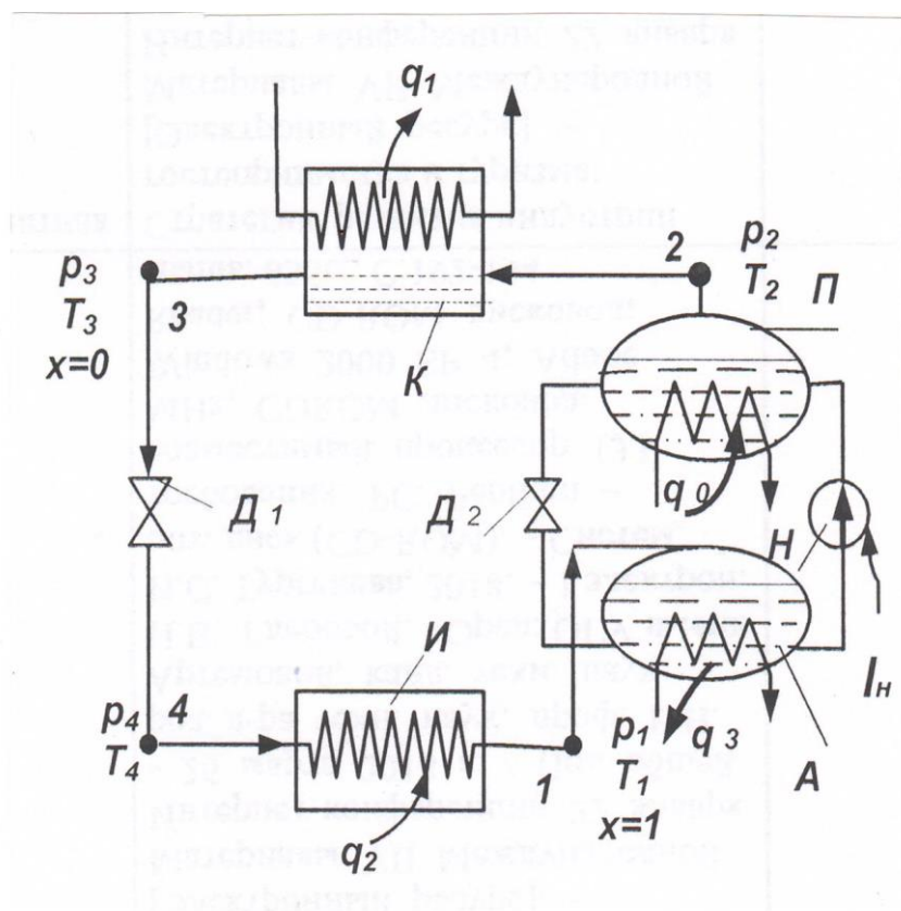
Рисунок 1 – Цикл парокompрессионной холодильной установки
