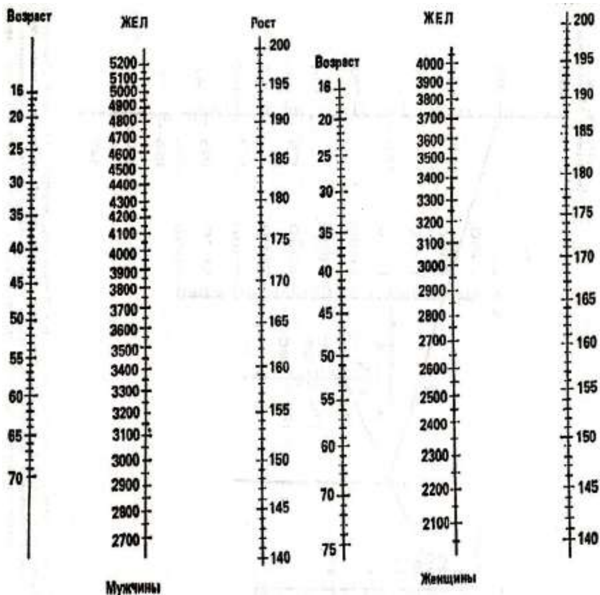
Рисунок 7. Номограмма для определения должной жизненной емкости легких в зависимости от роста и возраста
