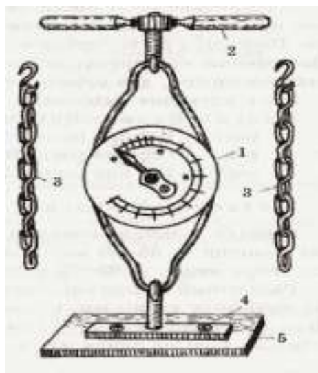
Рисунок 1. Динамометр становой: 1 – динамометр; 2 – рукоятка с крюком; 3 – цепь; 4 – планка с крюком; 5 – доска для закрепления планки с крюком
