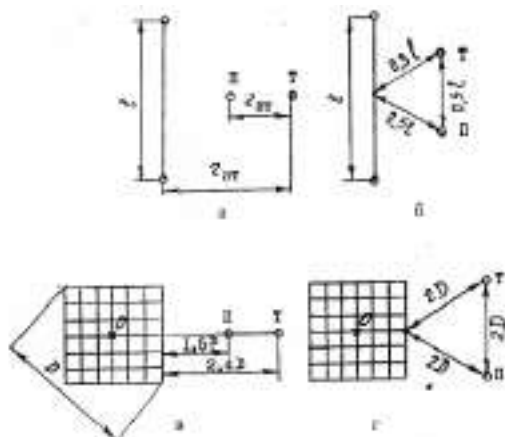
Рис. 6.4. Схемы расположения электродов II и Т при измерении сопротивления заземлителей: а – однолучевая (при l \leq 6 м r_{II} = 40 м, r_{TT} = 15 м; при l > 6 м r_{II} = 6 м, r_{TT} = 0,5 м); б – двухлучевая; в, г – соответственно однолучевая и двухлучевая для сложного заземления в виде контура
