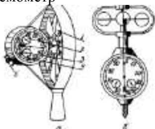
Рис. 1.4. Анемометры: а – крыльчатый, б – чашечный 1 – крыльчатка, 2, 3, 4 – счетно-отсчетный механизм, датчик и кабели оборотов, 5 – арретир
