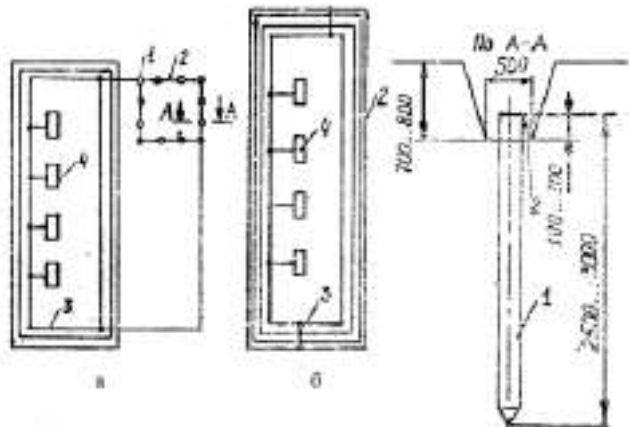
Рис. 6.2. Конструкция защитного заземления: а – вертикальный; б – контурный; 1 – вертикальный заземлитель; 2 – горизонтальный заземлитель; 3 – вертикальные проводники; 4 – электроустановка
