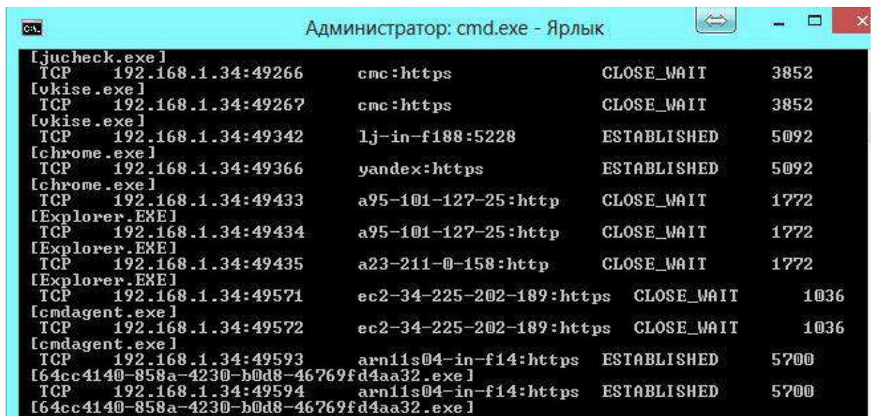
Рисунок 3 – результат сетевой статистики
