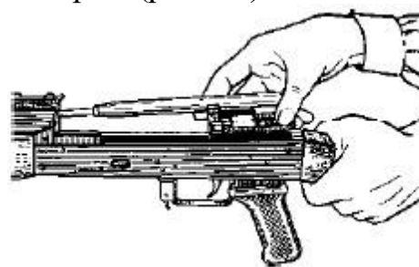
Рис. 15. Отделение затворной рамы с затвором
