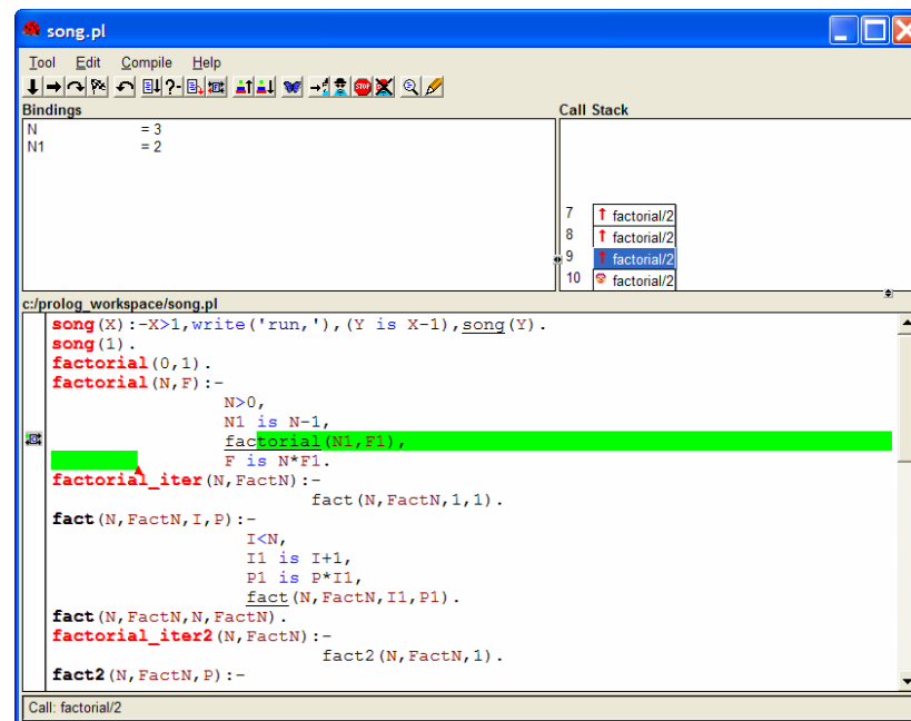
Рисунок 1.8 – Результат трассировки
