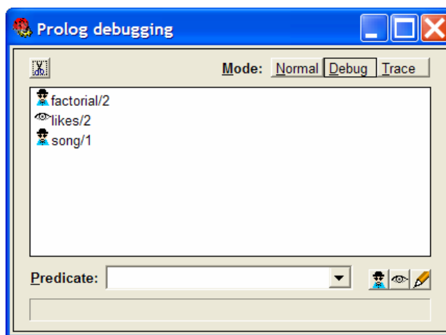
Рисунок 1.5 – Режим трассировки
