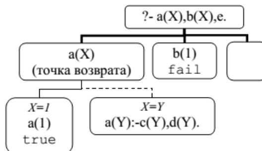
Рисунок 1.6 – Выполнение программы
