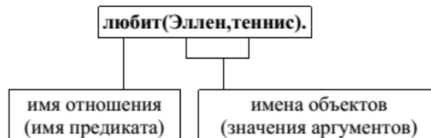
Рисунок 1.2 – Синтаксис Пролог
