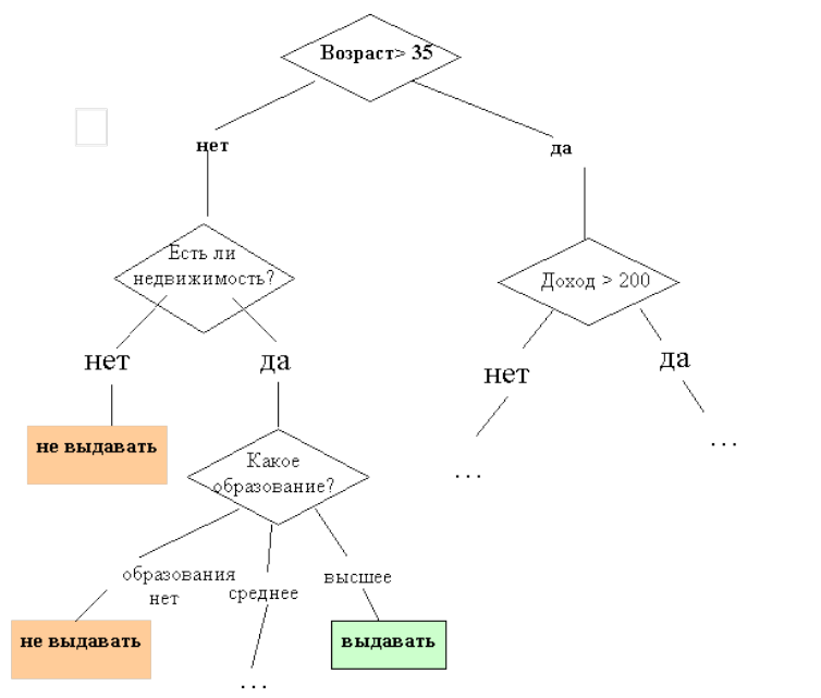
Рисунок 6.2 -Дерево решений "Выдавать ли кредит?"
