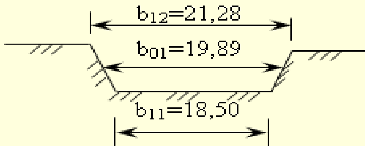
Рисунок 9 Котлован под здание
