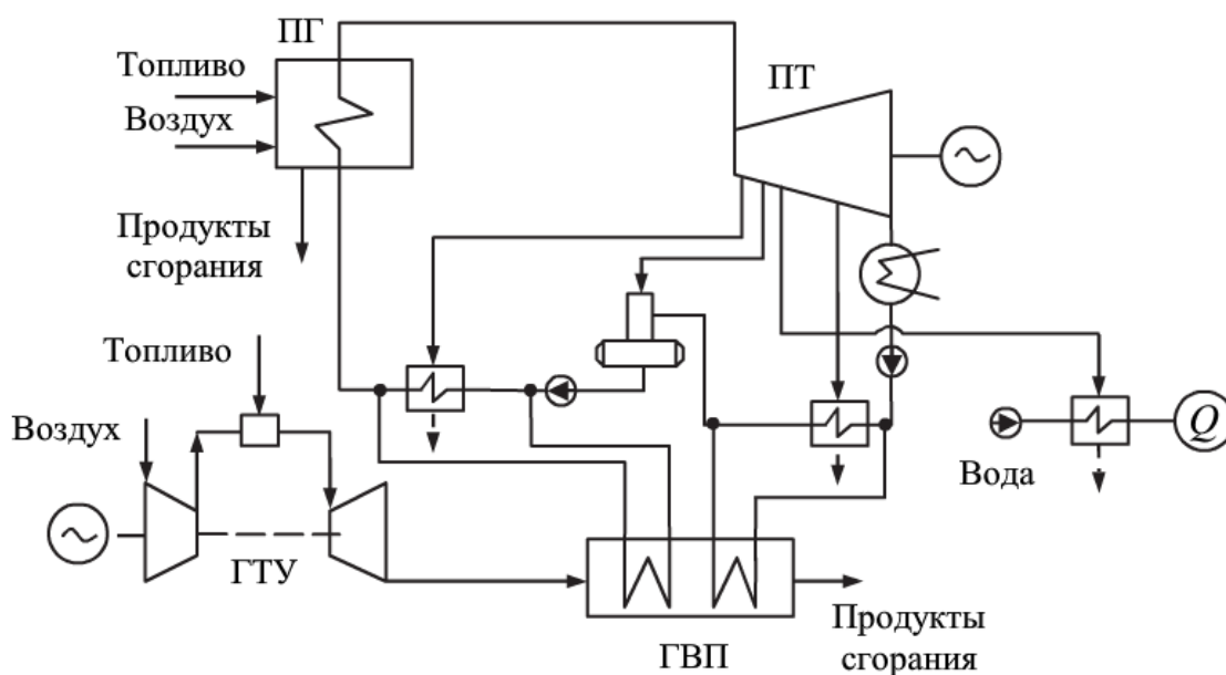
Рисунок 3.4 – Принципиальная тепловая схема ПГУ с ГВП: ПГ – парогенератор; ГВП – газовой водяной подогреватель
