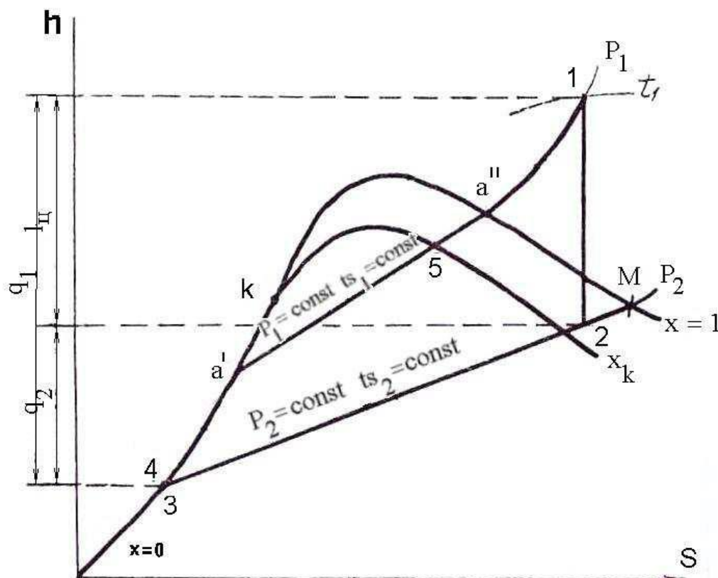
Рисунок 8.3 – h - s диаграмма цикла Ренкина
