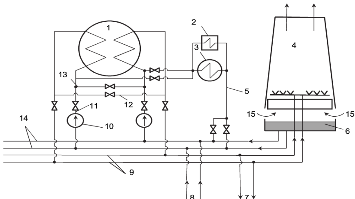
Рисунок 4.3 – Схема оборотного водоснабжения с градирней:
